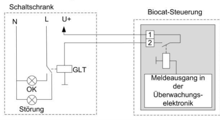
Beispielbeschaltung 2: Einbindung in GLT (Digital-Eingang)
