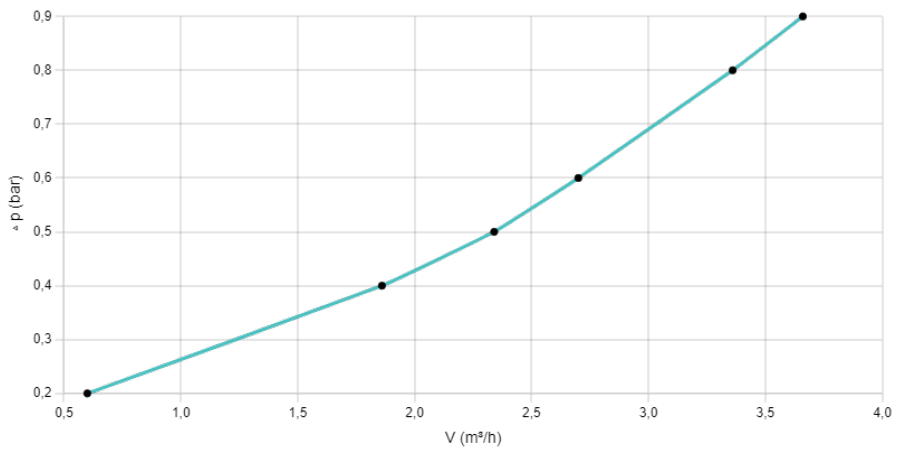
Volumenstrom KLS 3000-C
