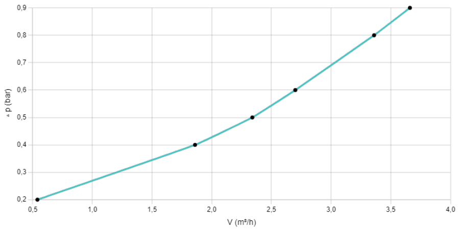
Volumenstrom KLS 4000-C
