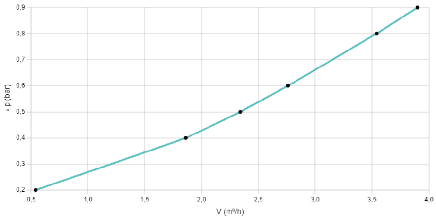
Volumenstrom KS 4000-C
