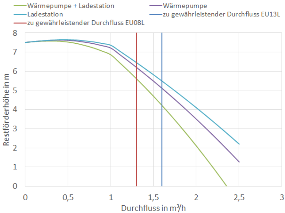
Abbildung 34: Restförderhöhe
