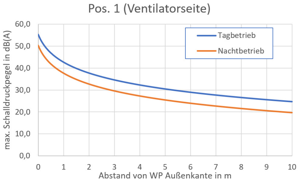
Abbildung 35: Schalldruckpegel EU08L, Vorderseite, freistehend
