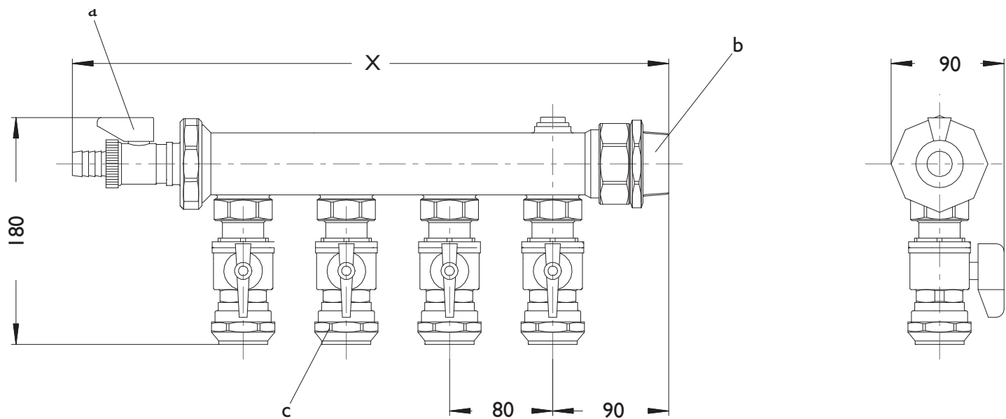
Massbild 3, 4fach
