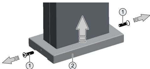
4. Ábra: A burkolat meglazítása
