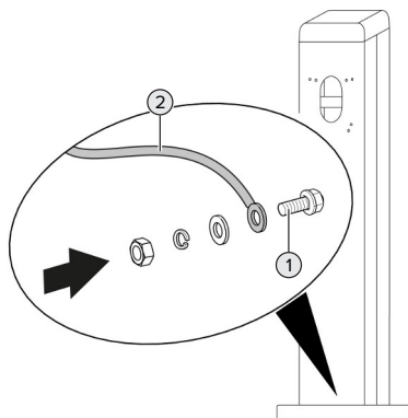
Fig. 3 : Mise à la terre du produit
