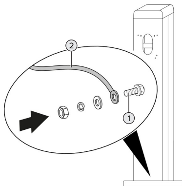
Fig. 3: Messa a terra del prodotto
