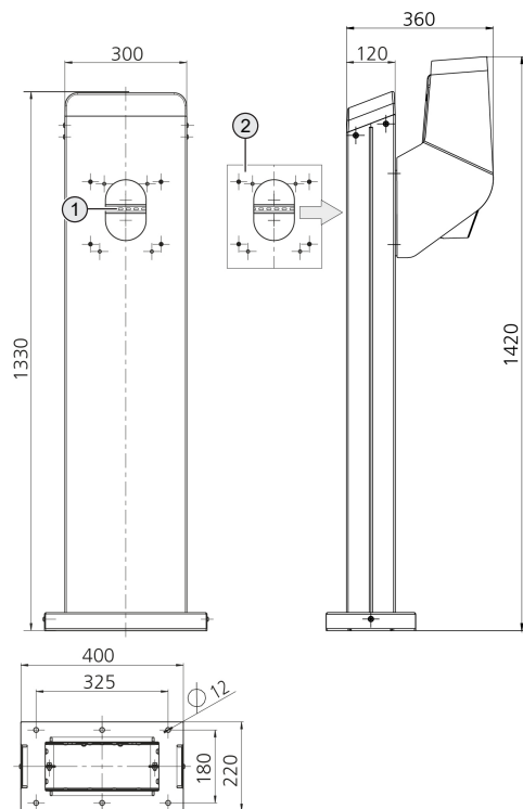
2. Ábra: Méretek [mm]
