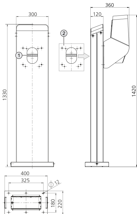
Abb. 2: Abmessungen [mm]
