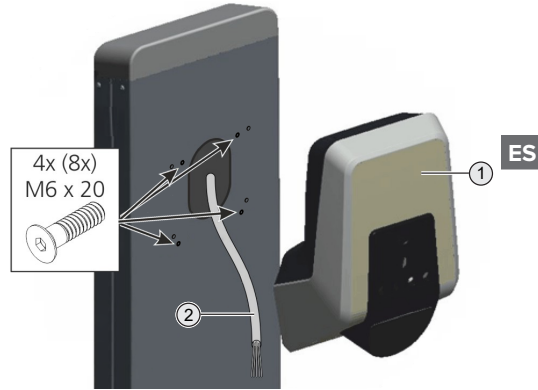
Fig. 6: Montaje del AMTRON®
