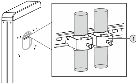
5. Ábra: A tápvezeték húzásmentesítése
