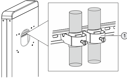
Fig. 5: Descarga de tracción de la línea de alimentación
