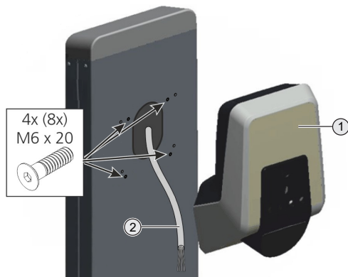
Fig. 6: Montaggio dell'AMTRON®
