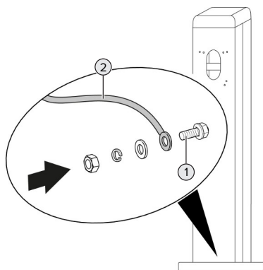
Fig. 3: Puesta a tierra del producto
