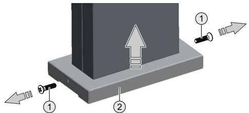
Abb. 4: Abdeckung lösen
