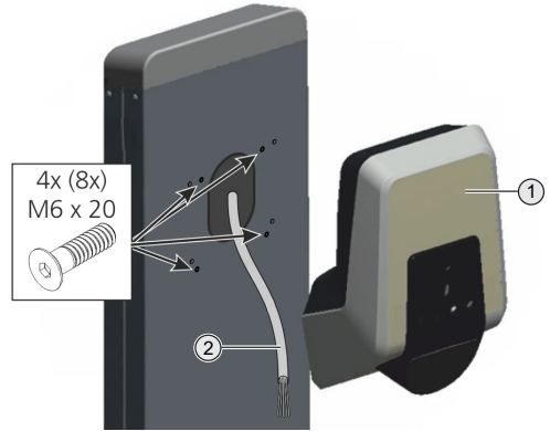
6. Ábra: Az AMTRON® felszerelése
