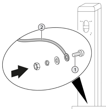
3. Ábra: A termék földelése
