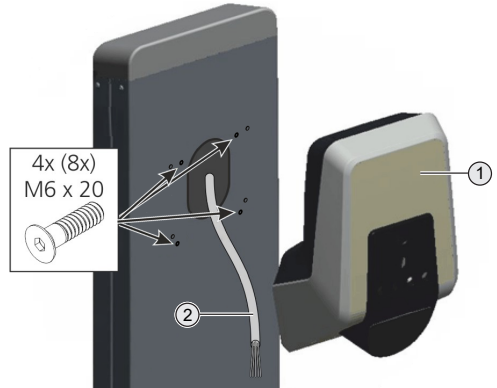
Abb. 6: AMTRON® montieren
