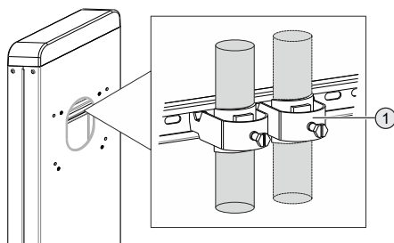
Afb. 5: Trekcontlasting van de voedingsleiding
