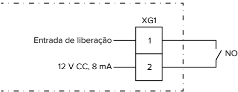
Fig. 17: Esquema de princípio: Entrada de liberação
