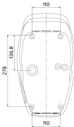
Εικ. 8: Διαστάσεις διάτρησης [mm]
