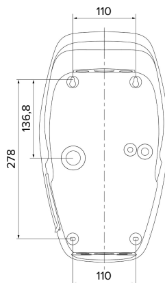
Fig. 8: Boremål [mm]
