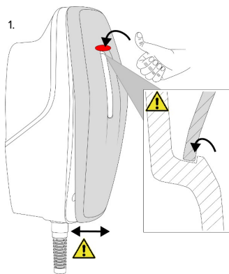
20. Ábra: Az előlap felhelyezése - 1
