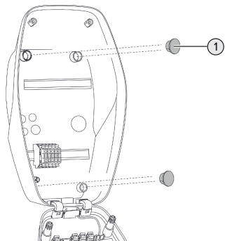
Kuva 9: Sulkutulpat
