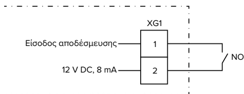
Εικ. 17: Διάγραμμα συνδεσμολογίας: Είσοδος αποδέσμευσης
