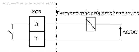
Εικ. 12: Διάγραμμα συνδεσμολογίας: Σύνδεση εξωτερικού ενεργοποιητή ρεύματος λειτουργίας
