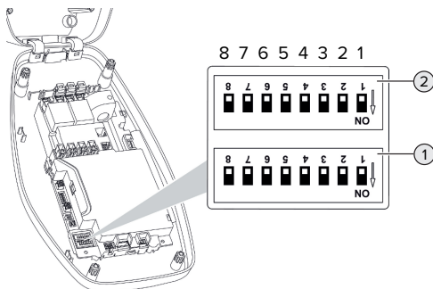
Fig. 13: DIP-kontakter (udleveringstilstand)
