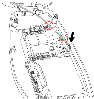
Ilustr. 14: Przyłącze wejścia Downgrade
