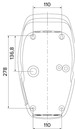
8. Ábra: Furatméretek [mm]
