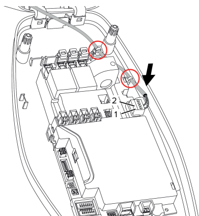
Fig. 16: Tilkobling frigivelsesindgang
