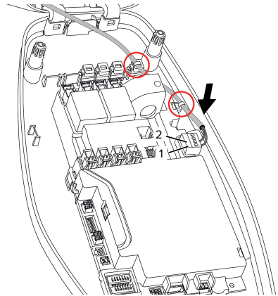
Fig. 16 : Raccordement de l'entrée de validation
