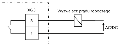
Ilustr. 12: Schemat blokowy: podłączenie zewnętrznego wyzwalacza prądu roboczego
