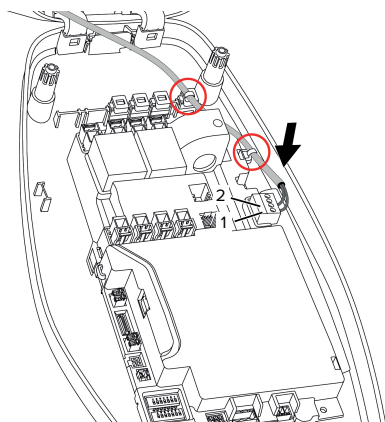
Kuva 16: Liitäntä vapautustulo
