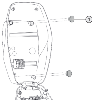
Fig. 9: Lukkepropper
