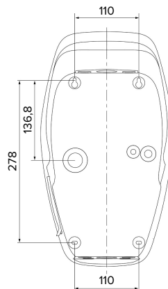
Fig. 8: Dimensioni dei fori [mm]
