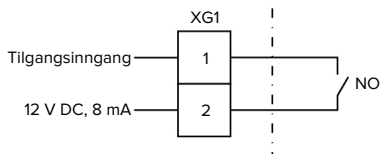
Fig. 17: Prinsipielt koblingsskjema: Tilgangsinngang
