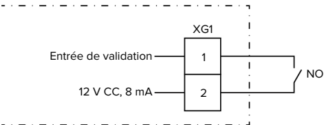
Fig. 17 : Schéma de principe : Entrée de validation
