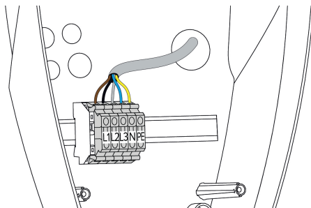
Pav. 10: Maitinimo įtampos jungtis
