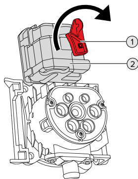
Εικ. 24: Χειροκίνητη απασφάλιση του βύσματος φόρτισης
