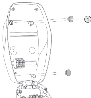
Abb. 9: Verschlussstopfen
