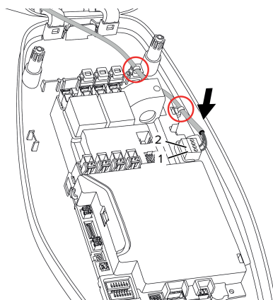
Εικ. 16: Δύνδεση εισόδου αποδέσμευσης
