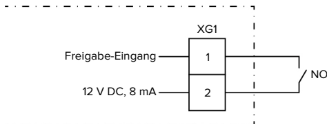
Abb. 17: Prinzipschaltbild: Freigabe-Eingang
