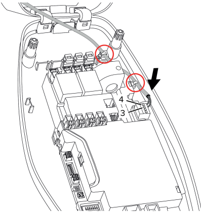
Abb. 14: Anschluss Downgrade-Eingang
