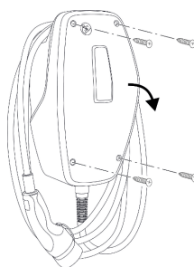
Fig. 6: Åpne produktet
