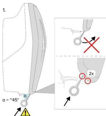
sl. 4: Odstranitev sprednjega pokrova – 1
