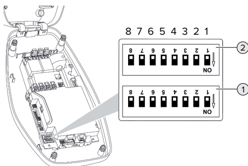
Afb. 13: Dipschakelaar (uitleveringstoestand)
