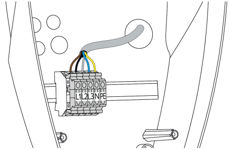
10. Ábra: Feszültségellátás csatlakoztatása
