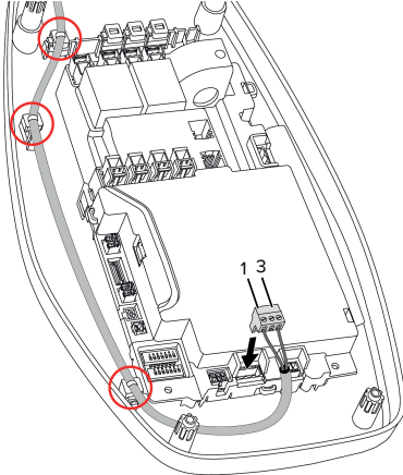
Kuva 11: Työvirtalaukaisijan liitäntä
