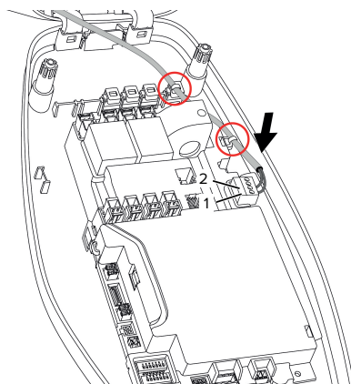
Fig. 16: Collegamento ingresso di abilitazione
