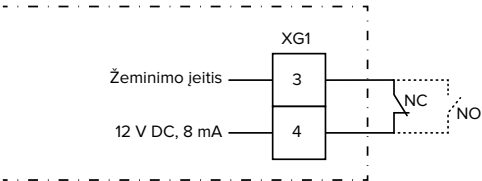
Pav. 15: Principinė sujungimo schema: išorinio jungimo kontakto jungties prijungimas (standartinis nustatymas: NO)
