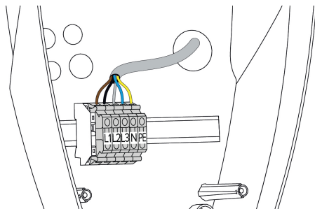
Fig. 10: Tilkobling spenningstilførsel
