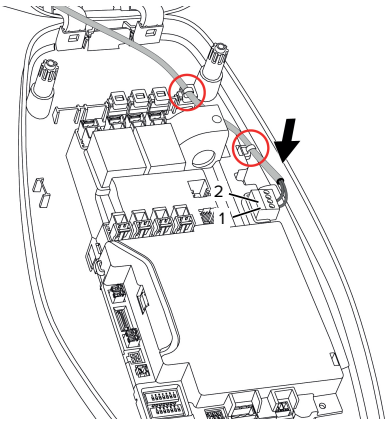
Fig. 16: Conexión entrada de habilitación
