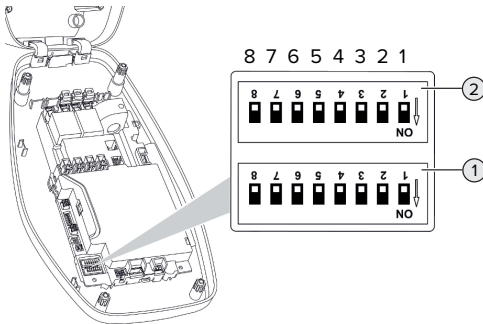
Fig. 13: DIP-brytare (leveranstillstånd)
