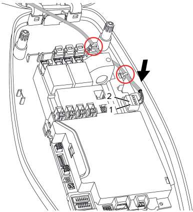
Fig. 16: Ligação da entrada de liberação
