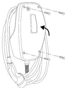
Εικ. 18: Κλείσιμο του προϊόντος
