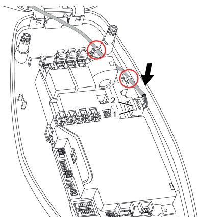
Fig. 16: Tilkobling tilgangsinngang
