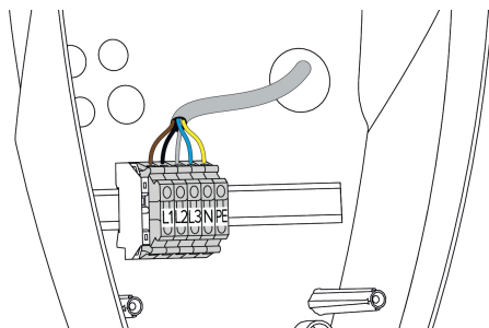
Abb. 10: Anschluss Spannungsversorgung
