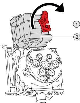
sl. 24: Ročna sprostitelj polnilnega vtiča
