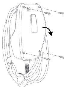
Abb. 6: Produkt öffnen
