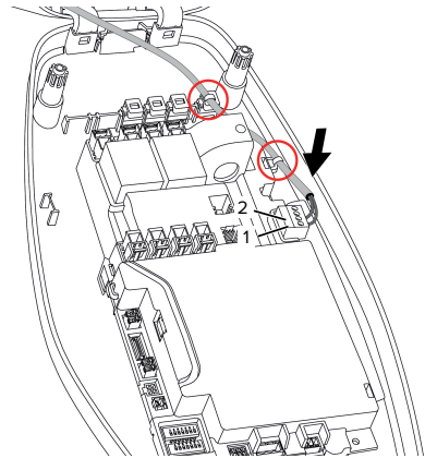
Afb. 16: Aansluiting vrijgave-ingang
