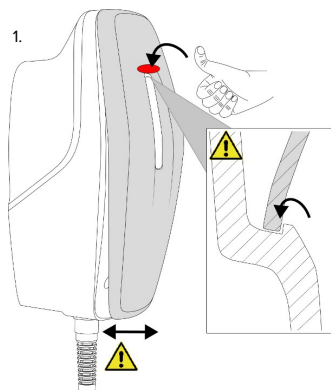
Afb. 20: Frontcover aanbrengen - 1
