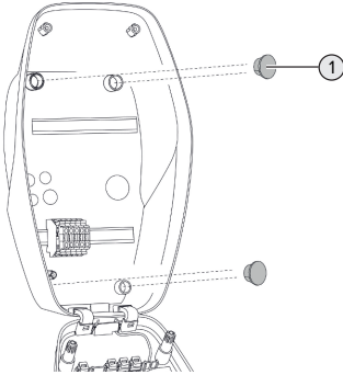
9. Ábra: Záródugók
