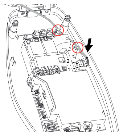
Fig. 16: Anslutning av aktiveringsingång
