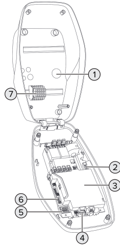
Kuva 3: Sisänäkymä (esimerkki)
