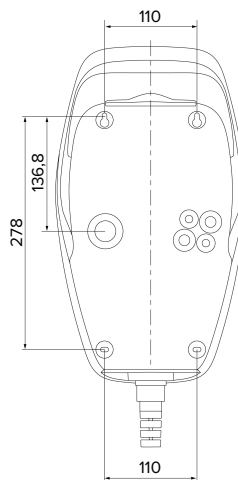
Ilustr. 7: Wymiary wiercenia [mm]
