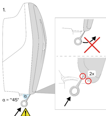
4. Ábra: Az előlap eltávolítása - 1
