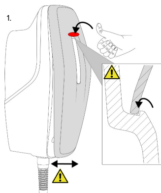
Εικ. 20: Τοποθέτηση του μπροστινού καλύμματος - 1
