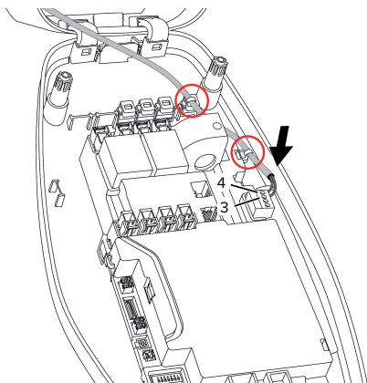
Fig. 14: Tilslutning downgrade-indgang
