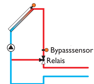
Beispielschemata für die verschiedenen Bypass-Varianten
