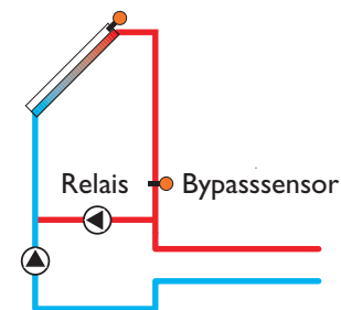
Beispielschemata für die verschiedenen Bypass-Varianten
