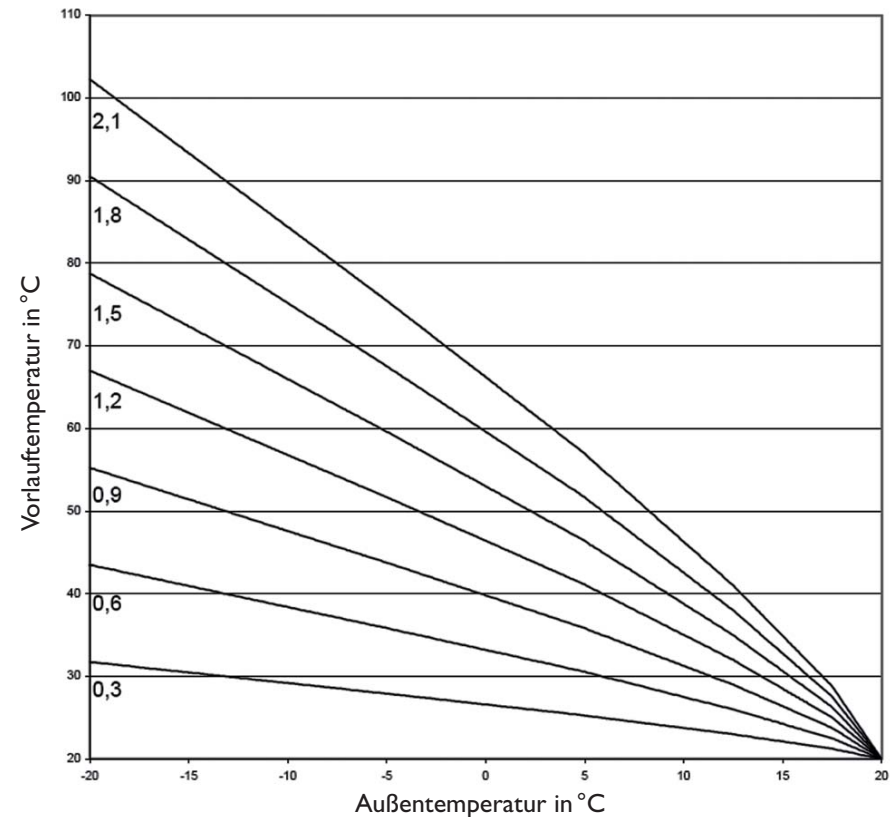
Heizkennlinien
