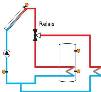
Variante Ventil
