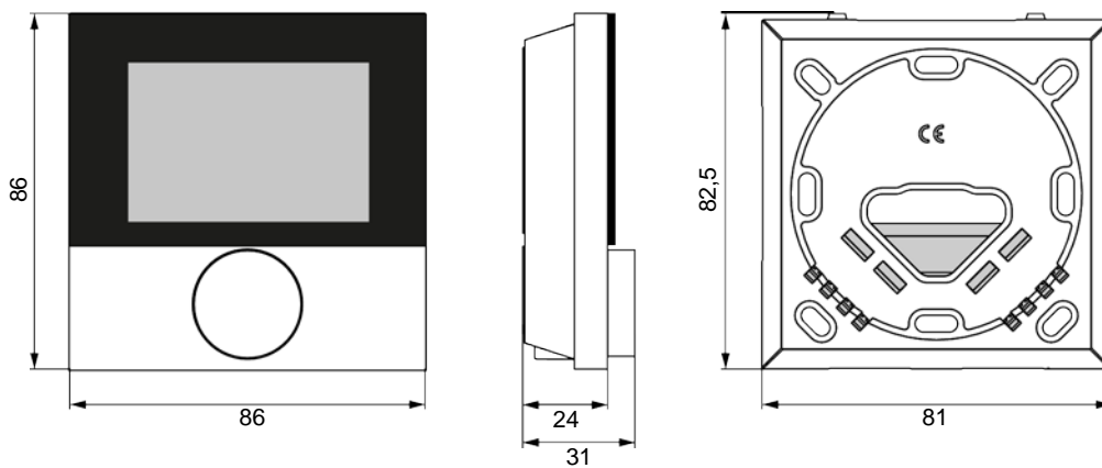
Abmessungen (alle Angaben in mm)
