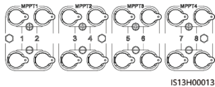
Abbildung 5-7 DC-Eingangsklemmen
