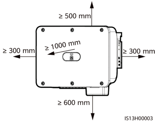
Abbildung 4-2 Montageabstände
