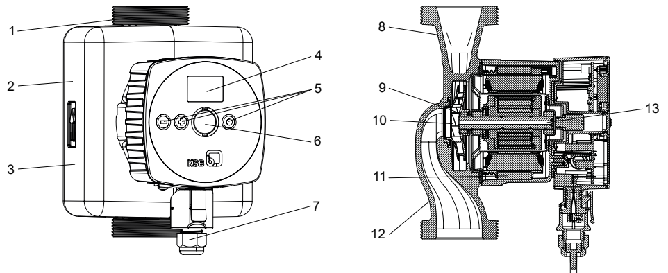
Abb. 2: Darstellung Pumpenaggregat
