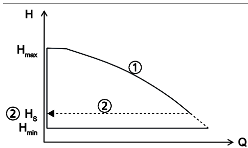
Abb. 9: Funktion Konstantdruckregelung
