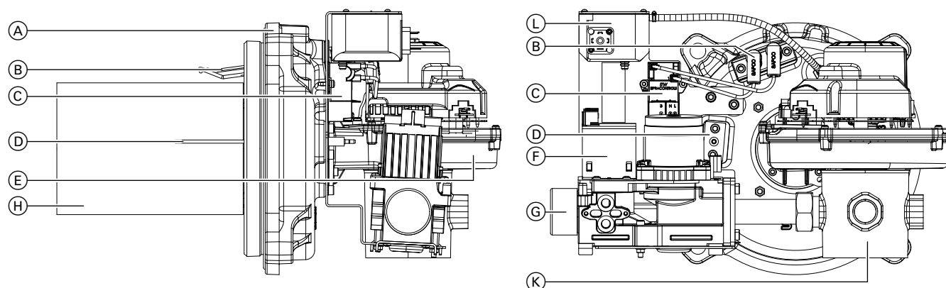
MatriX-Zylinderbrenner 120 bis 160 kW
