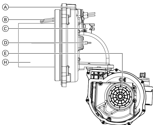
MatriX-Zylinderbrenner bis 80 kW
