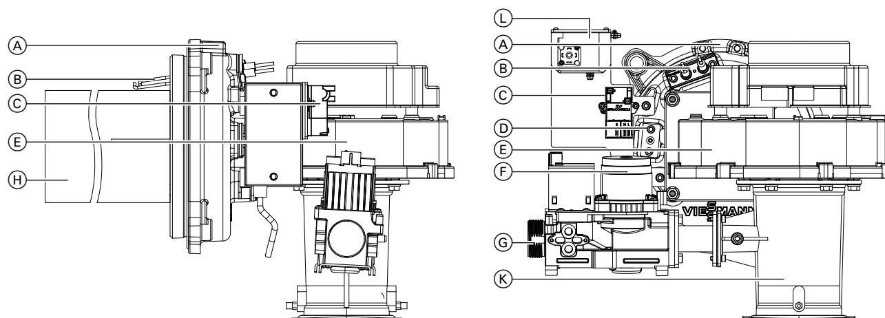
MatriX-Zylinderbrenner ab 200 kW
