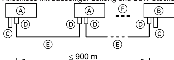
Abb. 5 Verlegeabstand \leq 900 m (mit LON-Stecker)
