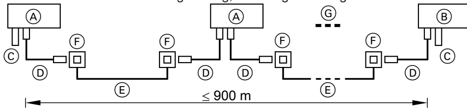
Abb. 6 Verlegeabstand \leq 900 m (mit LON-Anschlussdosen)
