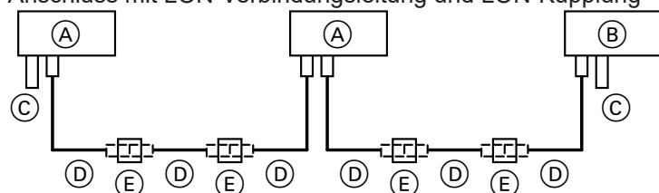
Abb. 4 Verlegeabstand 7 bis 21 m
