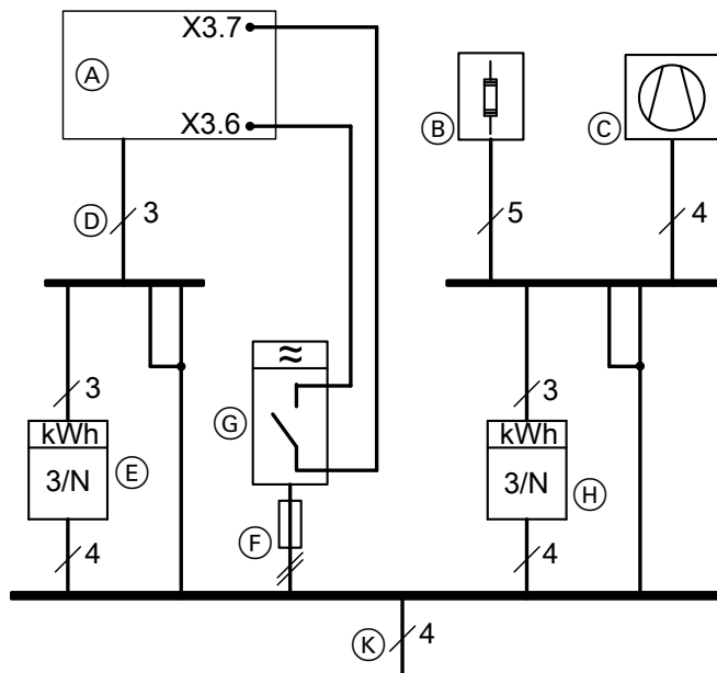
Abb. 38 Darstellung ohne Sicherungen und ohne FI-Schutzschalter
