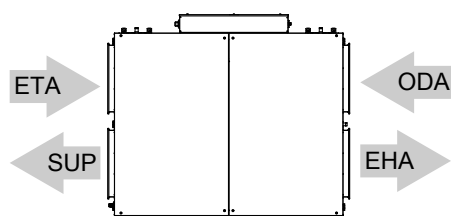
Abb. 1 Typ 1000/1500/2000/3000S-L
