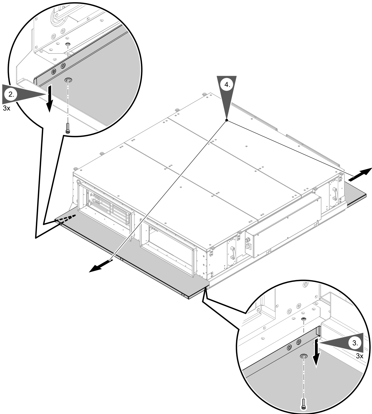
Abb. 65 Beispiel: Typ 1500S
