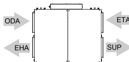
Abb. 2 Typ 1000/1500/2000/3000S-R
