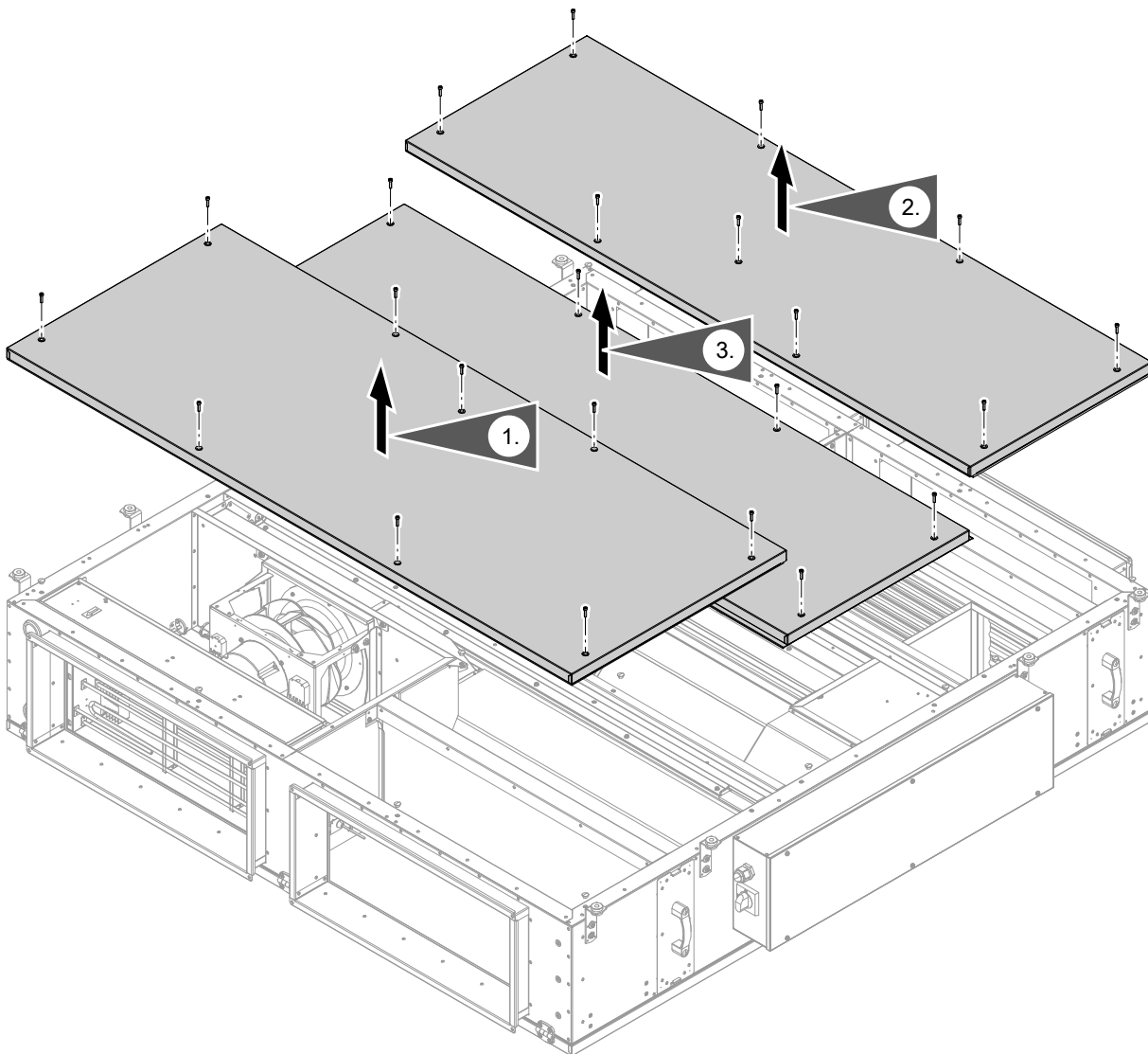
Abb. 63 Beispiel: Typ 1500S
