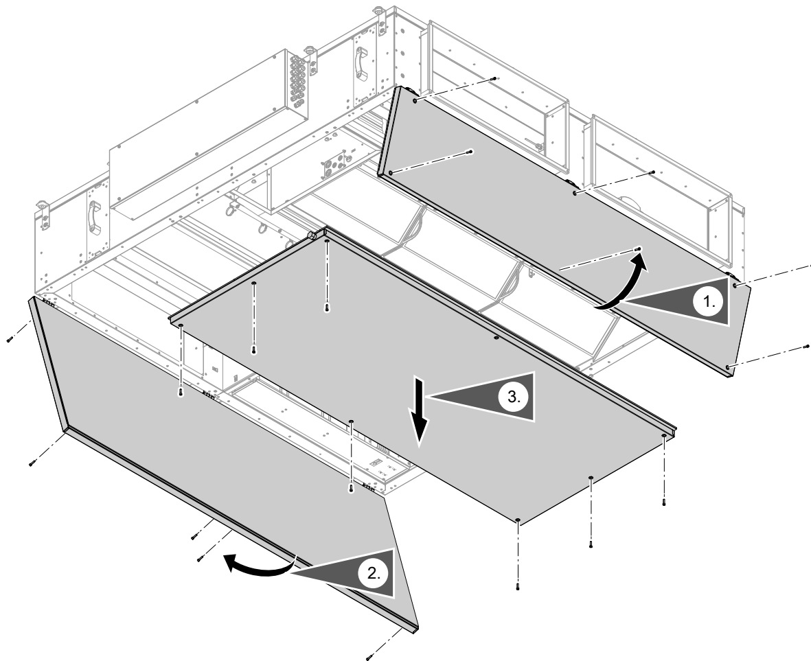
Abb. 64 Beispiel: Typ 1500S
