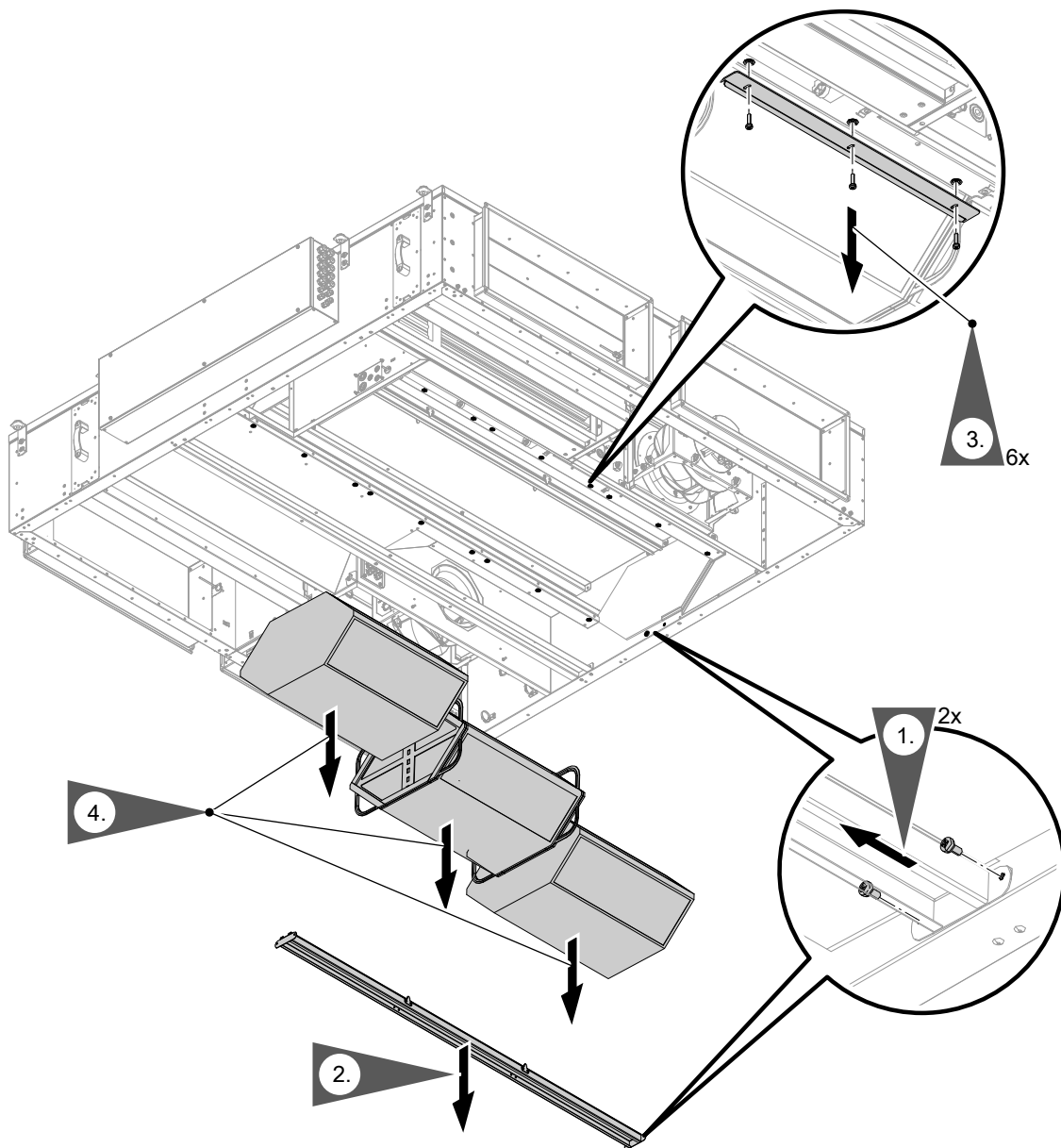
Abb. 67 Beispiel: Typ 1500S
