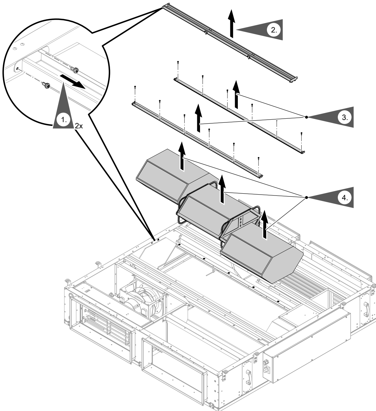
Abb. 66 Beispiel: Typ 1500S
