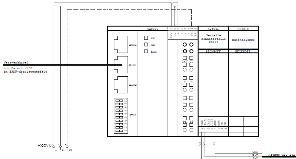
Abb. 1 Anschluss Gateway Modbus RTU 232
