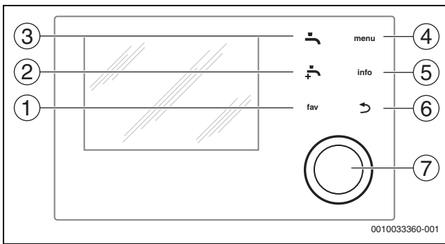
Bild 3 Bedienelemente
