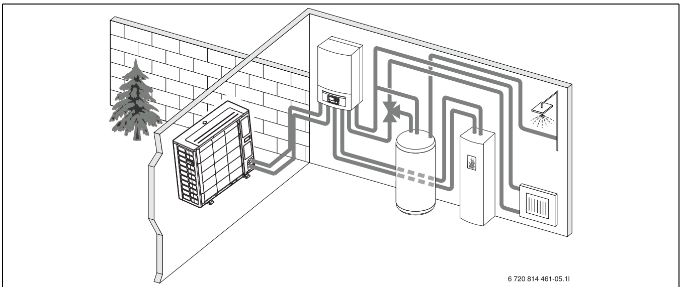
Bild 2 Wärmepumpe Außeneinheit, Inneneinheit IDUS B ohne elektrischen Zuheizter, externer Warmwasserspeicher und externer Zuheizter
