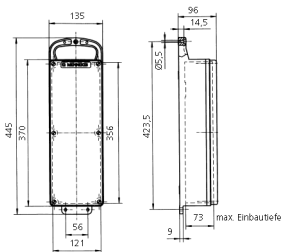
Zeichnung 5 MB 44 Maße in mm
