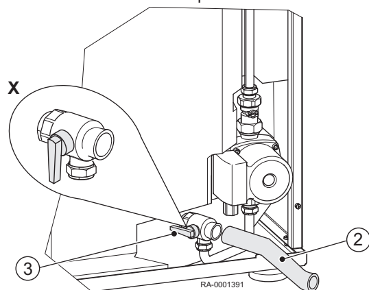
Abb.5 Entleeren des Speichers
