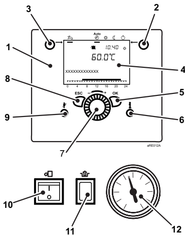
Abb.2 Bedienelemente
