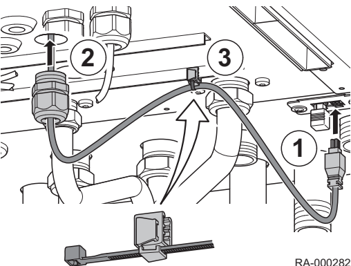
Abb.48 Verbindung mit L-Bus-Adapter
