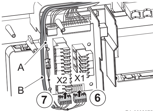
Abb.49 Anschluss an der Anschlussleiterplatte CB-28
