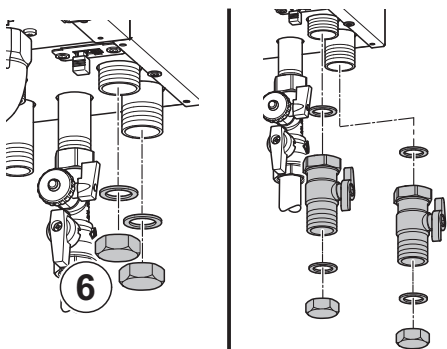
Abb.28 Anbringen der Verschlusskappen und Absperrhähne (optional)
