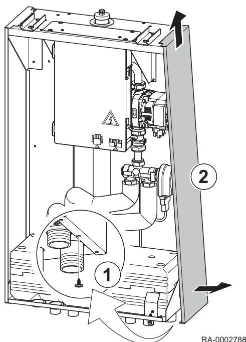
Abb.15 Entfernen der Regelungsbox (Darstellung ohne Gas- Brennwertkessel)
