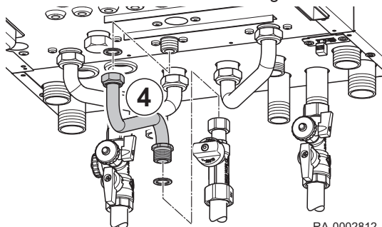
Abb.26 Installation der Gasleitung
