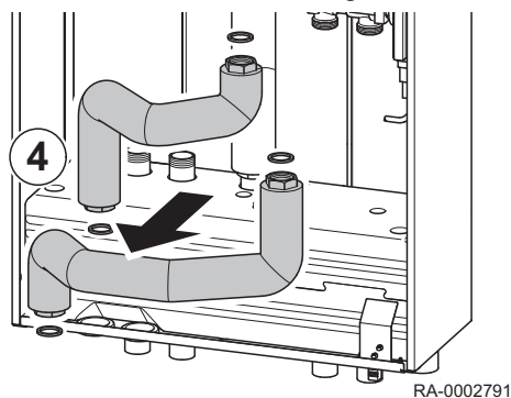
Abb.18 Entfernen der Rohrleitungen
