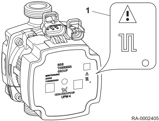
Abb.61 Statusanzeige Heizkreispumpe UPM4
