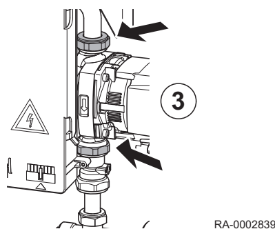
Abb.18 Entfernen der Rohrleitungen
