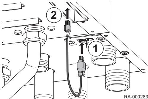
Abb.51 Verbindung mit L-Bus-Adapter
