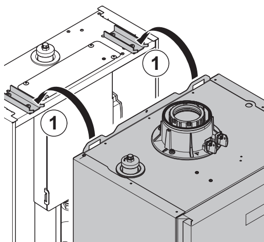
Abb.24 Montage des Gas-Brennwertkessels
