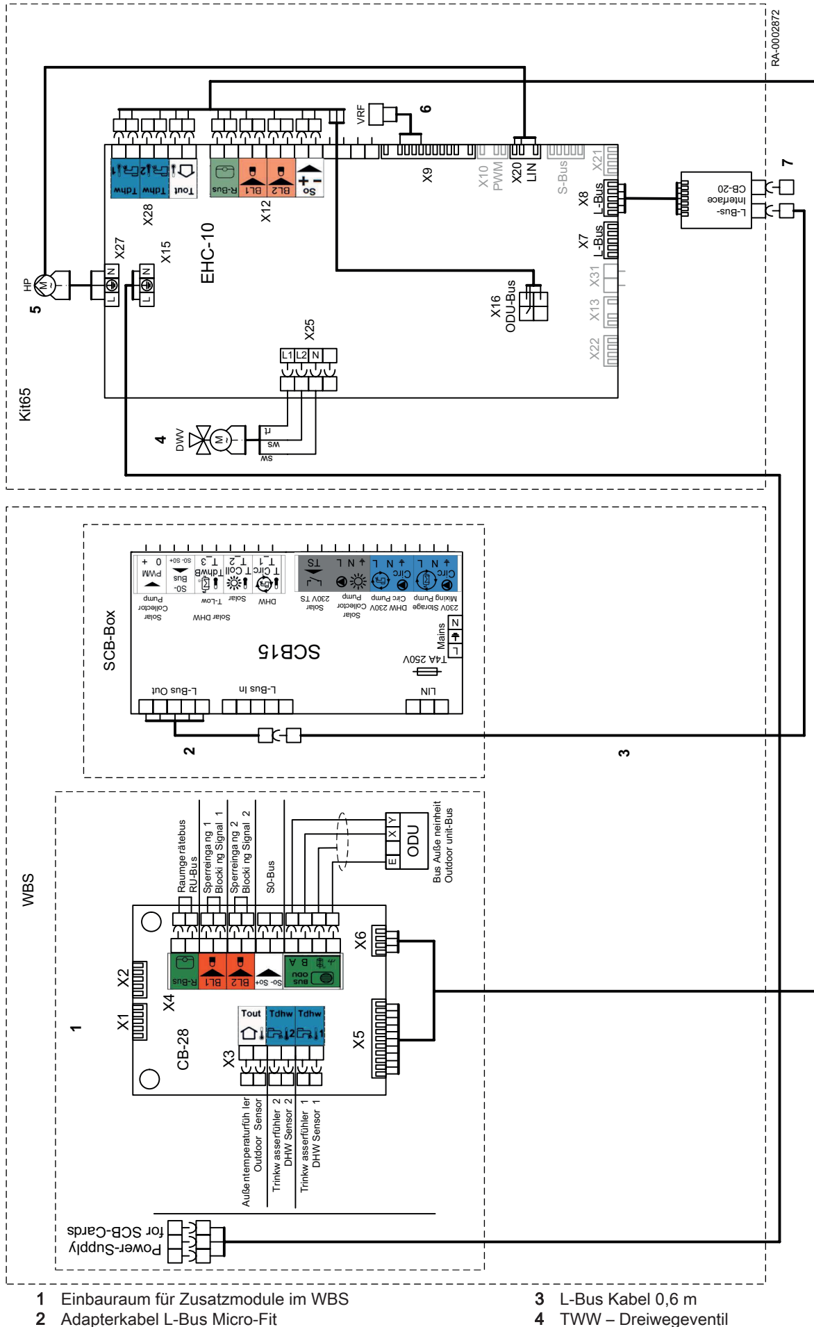
Abb.4 Schaltplan Kit 65 WBS mit SCB-15
