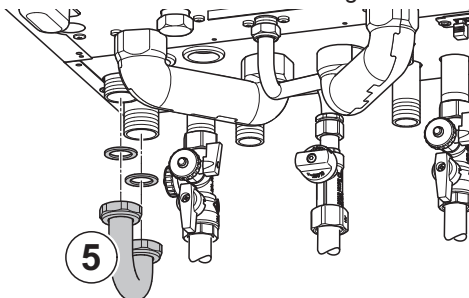
Abb.27 Installation der U-Rohrleitung
