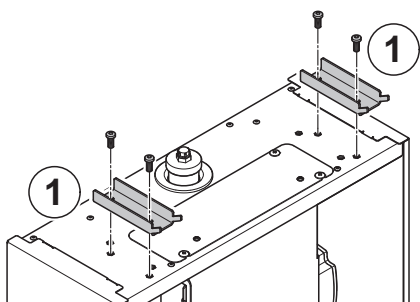
Abb.11 Montage der Kesselhalterungen
