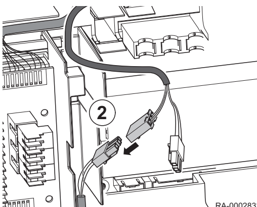
Abb.46 Verbindung der Netzanschlussleitung
