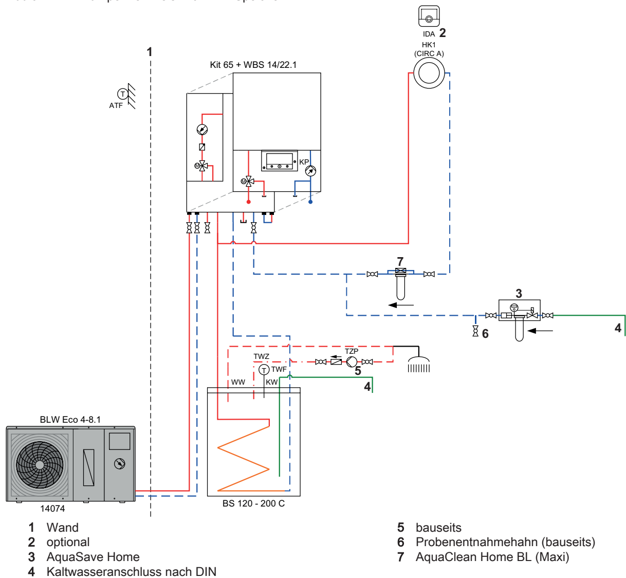
Abb.9 Ein Pumpenheizkreis mit TWW-Speicher
