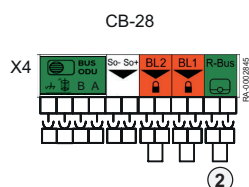
Abb.57 Anschließen eines Raumgerätes (an CB-28)
