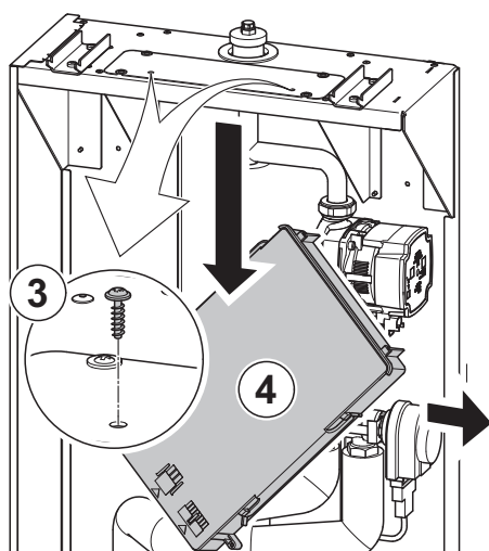
Abb.15 Entfernen der Regelungsbox (Darstellung ohne Gas- Brennwertkessel)
