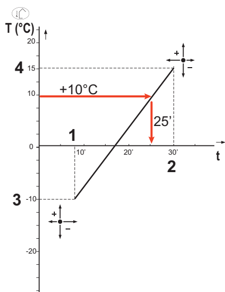
Abb.62 Zeitverzögerungskurve für das Einschalten des Zusatzheizung
