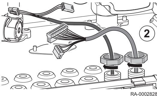
Abb.43 Kabelklammern
