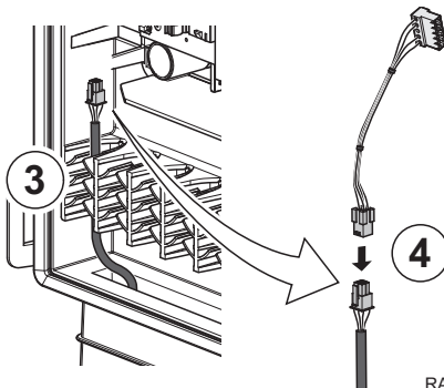
Abb.52 Anschluss an der Erweiterungsleiterplatte SCB-15
