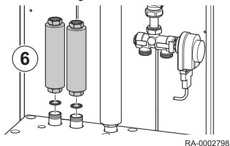
Abb.21 Drehen des Entlüftungsrohrs mit Pumpe
