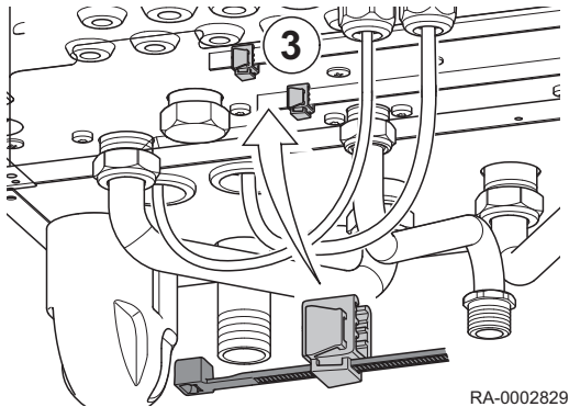
Abb.43 Kabelklammern
