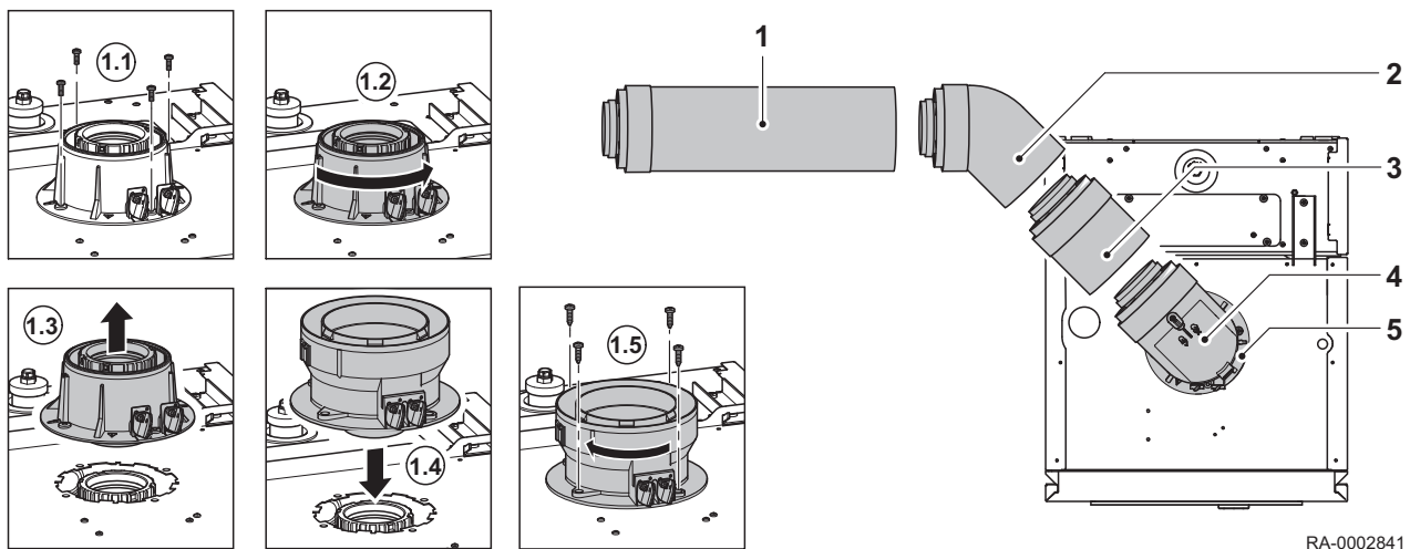
Abb.35 Abgasinstallation KAS 80 konzentrisch, zur Seite
