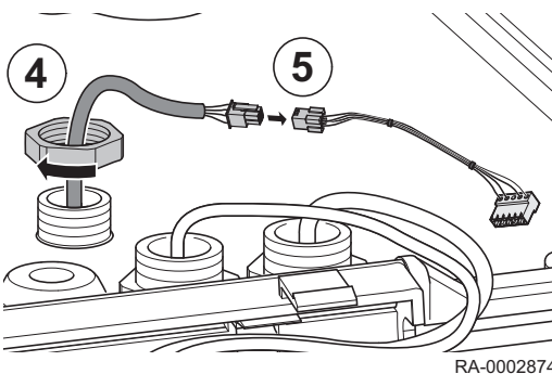
Abb.48 Verbindung mit L-Bus-Adapter
