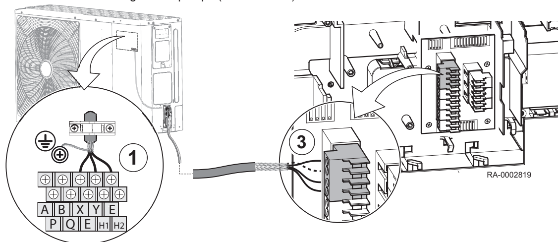
Abb.53 Busverbindung Wärmepumpe (Außeneinheit) / Gas-Brennwertkessel
