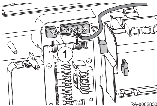
Abb.44 Verlegung der Verbindungskabel
