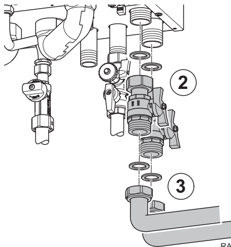
Abb.34 Wärmepumpe anschließen
