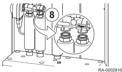
Abb.22 Verschraubungen festziehen
