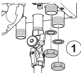
Abb.34 Wärmepumpe anschließen
