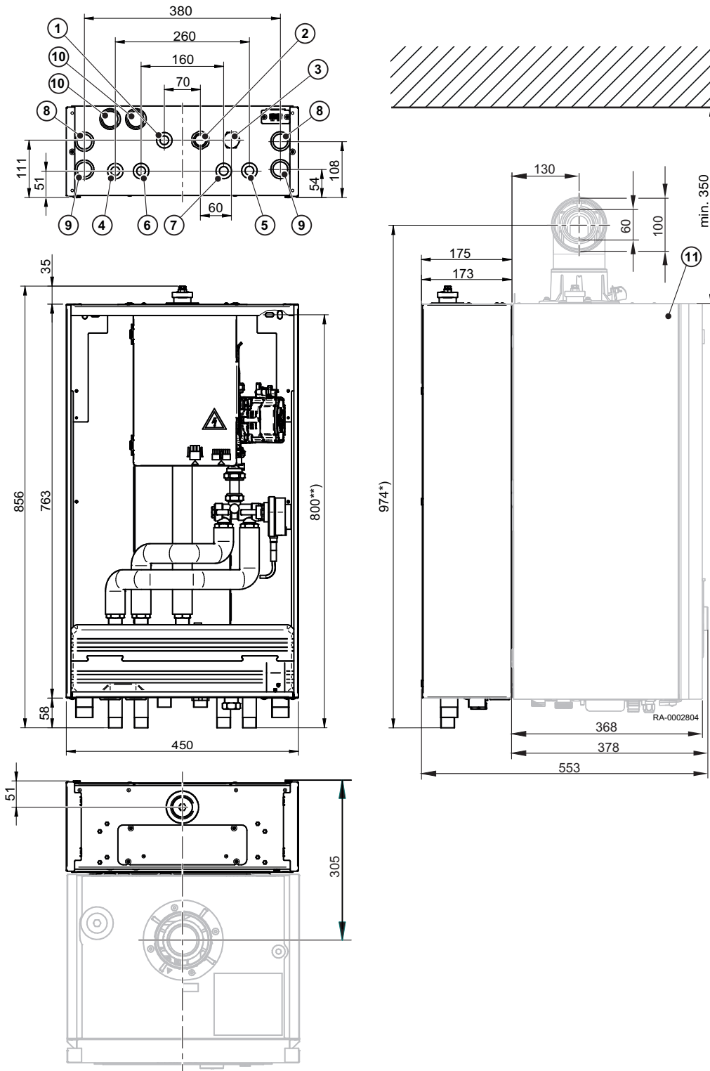
Abb.2 Abmessungen und Anschlüsse
