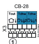
Abb.55 Außentemperaturfühler anschließen (an CB-28)
