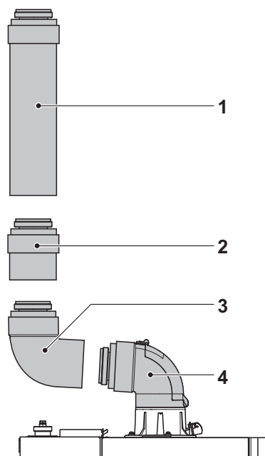
Abb.38 Abgasinstallation KAS 60 konzentrisch, nach oben
