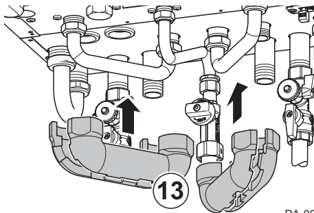
Abb.29 Montage der Dämmung
