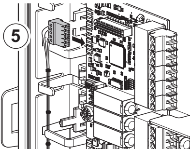
Abb.52 Anschluss an der Erweiterungsleiterplatte SCB-15
