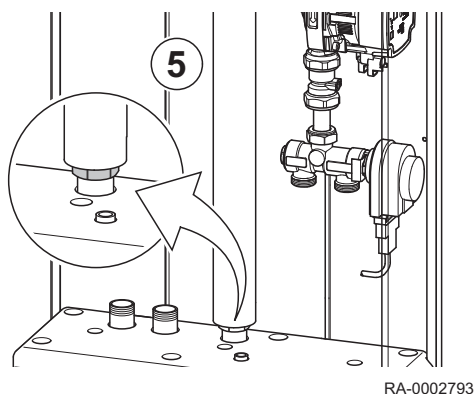
Abb.20 Installieren der geraden Rohrleitungen
