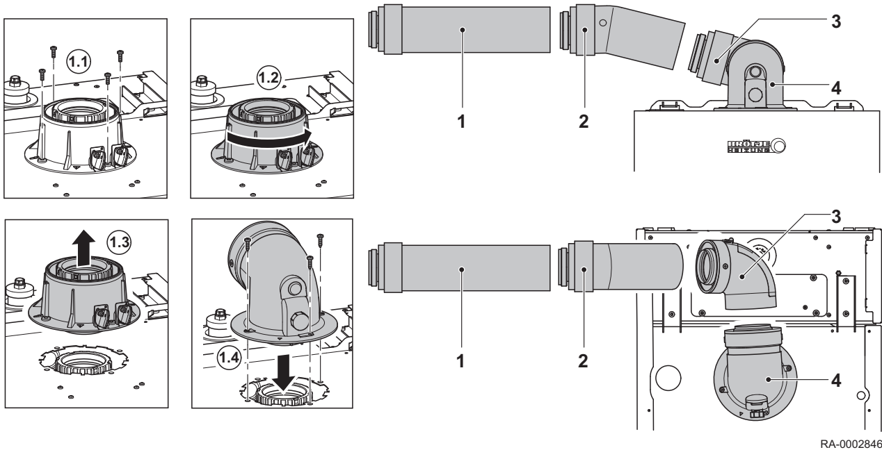
Abb.37 Abgasinstallation KAS 60 konzentrisch, zur Seite
