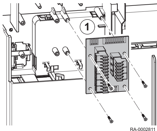
Abb.39 Montage CB-28
