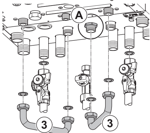
Abb.25 Installation der Rohrleitungen
