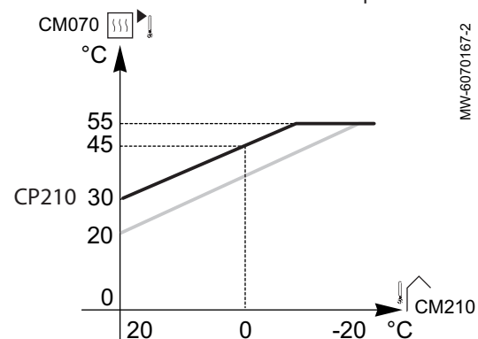
Abb.66 Heizkennlinie mit Grundtemperatur
