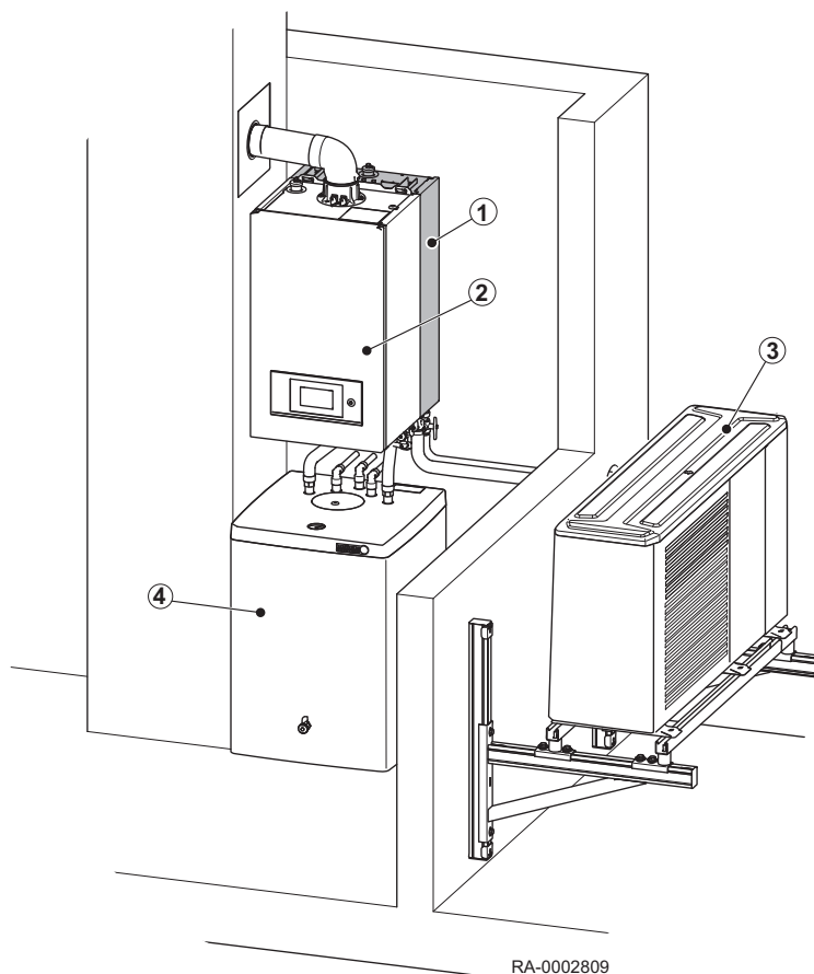
Abb.5 Kit 65 mit Kessel, Wärmepumpe und TWW-Speicher
