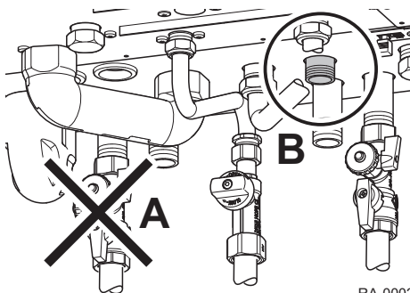
Abb.31 Anschluss Membran-Ausdehnungsgefäß
