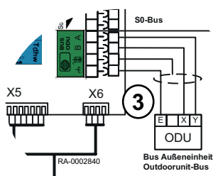
Abb.54 Klemme X10 "BUS ODU"
