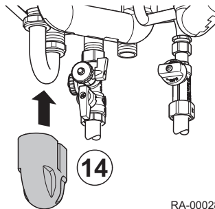
Abb.30 Montage der Dämmung
