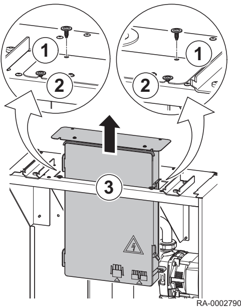
Abb.13 Entfernen der Regelungsbox
