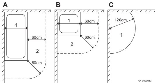
Abb.8 Abstände in Bad- und Duschräumen
