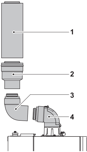
Abb.36 Abgasinstallation KAS 80 konzentrisch, nach oben
