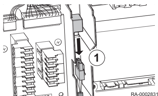
Abb.46 Verbindung der Netzanschlussleitung
