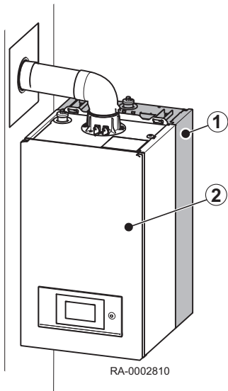
Abb.6 Kit 65 mit Kessel (Mindestausbau)
