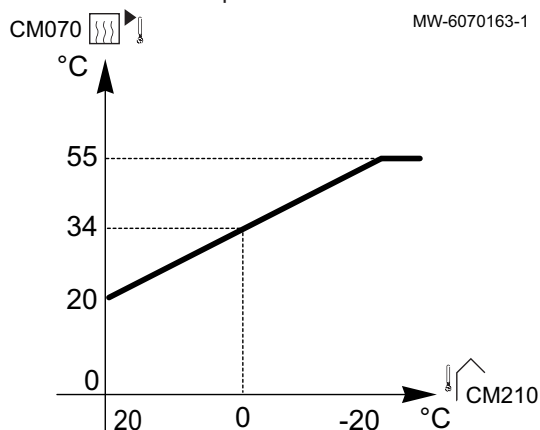
Abb.66 Heizkennlinie mit Grundtemperatur
