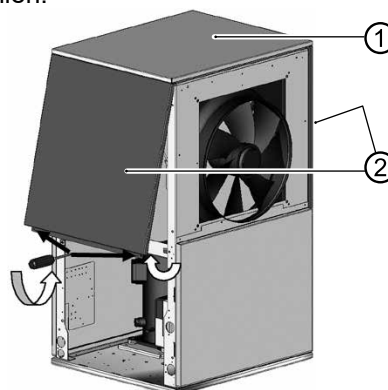
1 Gerätedeckel 2 obere Fassadierungen
