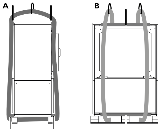
A Vorderansicht (Schaltkastenseite) B Seitenansicht 1
