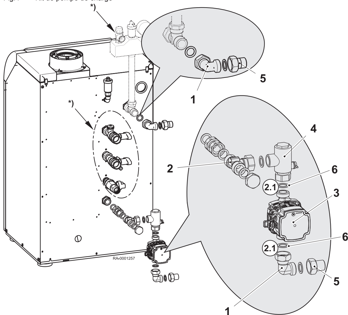
Fig.4 Kit de pompe de charge
