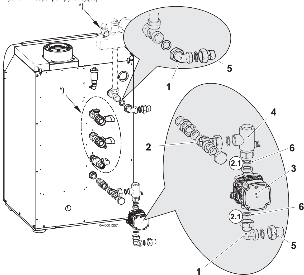
Rys.10 Zespół pompy ładującej
