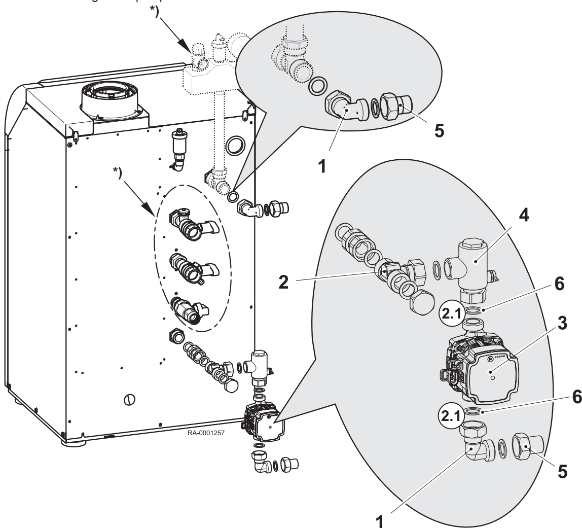
Abb.1 Montage Ladepumpenset
