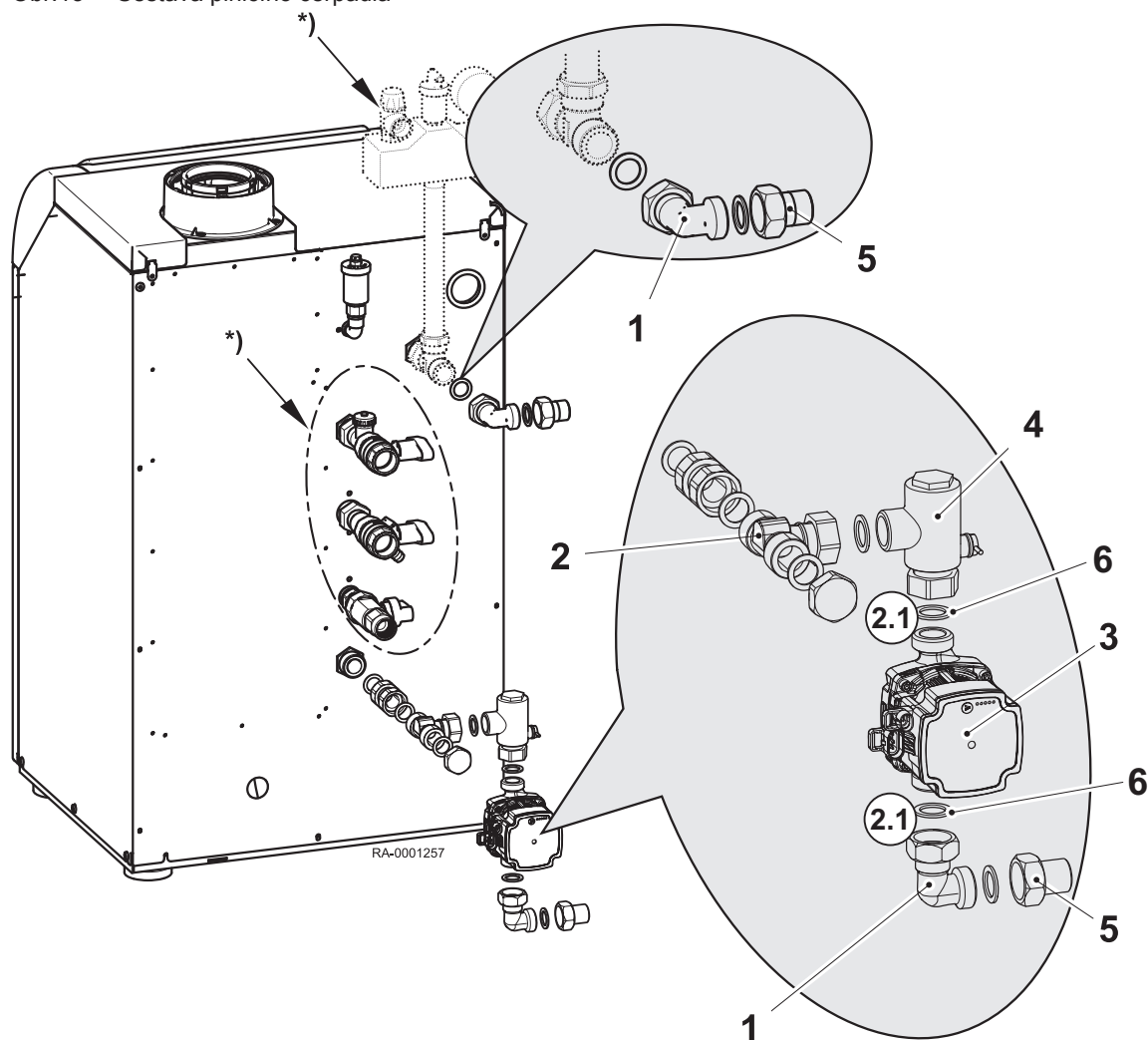
Obr.13 Sestava plnicího čerpadla
