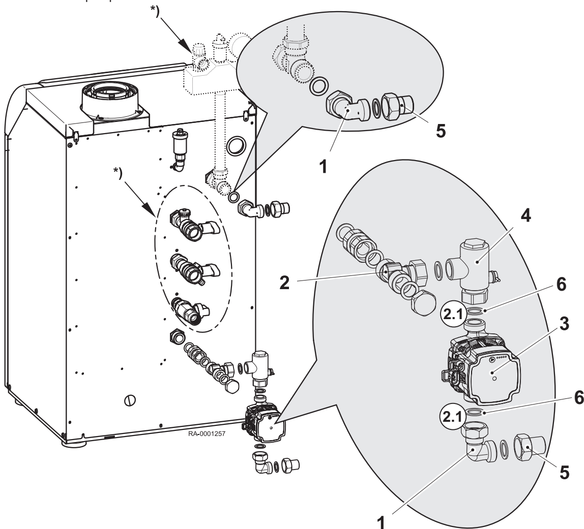
Afb.7 Laadpompset
