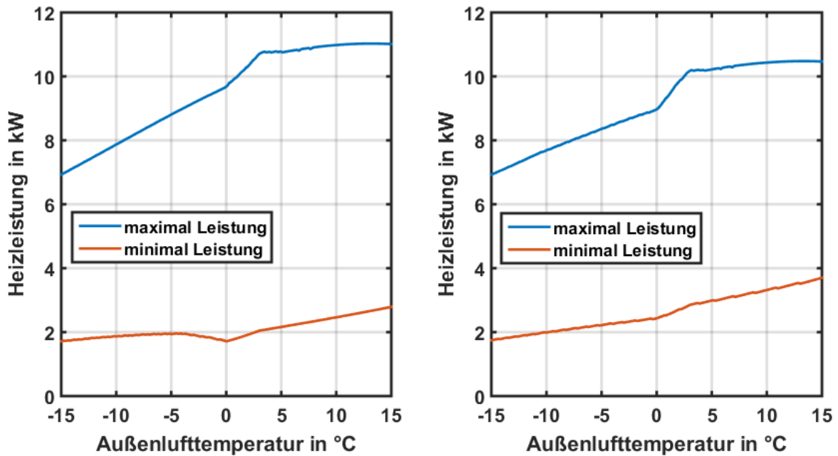
Abbildung 28: E08L bei 5K Spreizung (links: 35°C Vorlauftemperatur / rechts: 55°C Vorlauftemperatur)
