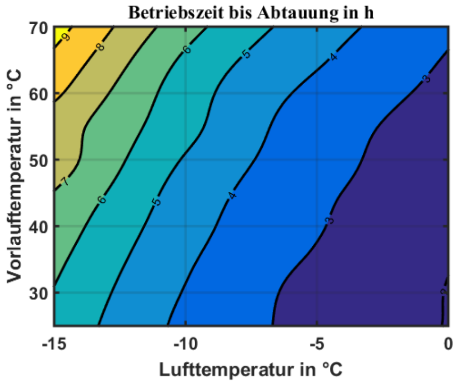
Abbildung 32: Betriebsdauer zwischen Abtauzyklen bei 6kW Heizleistung und 95% Luftfeuchte
