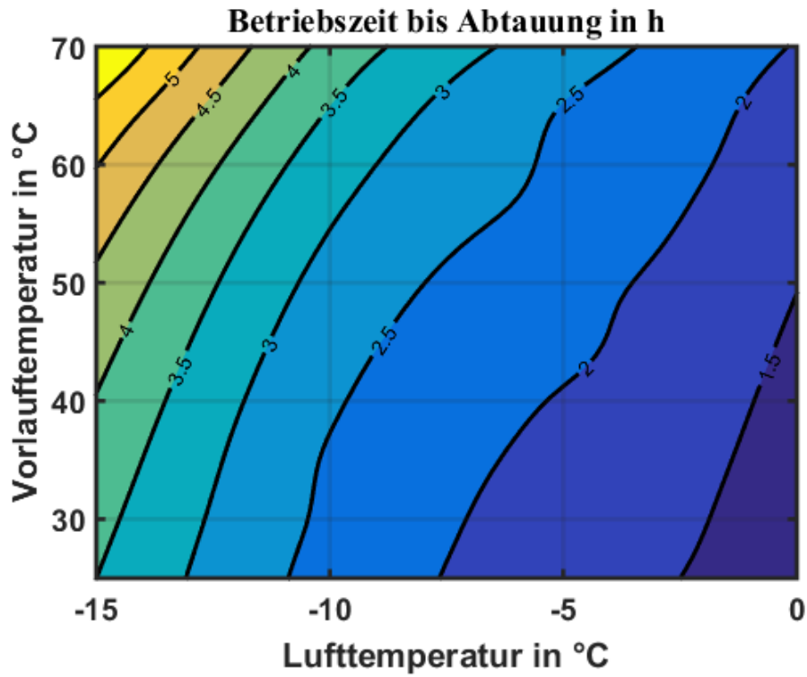
Abbildung 31: Betriebsdauer zwischen Abtauzyklen bei 9kW Heizleistung und 95% Luftfeuchte
