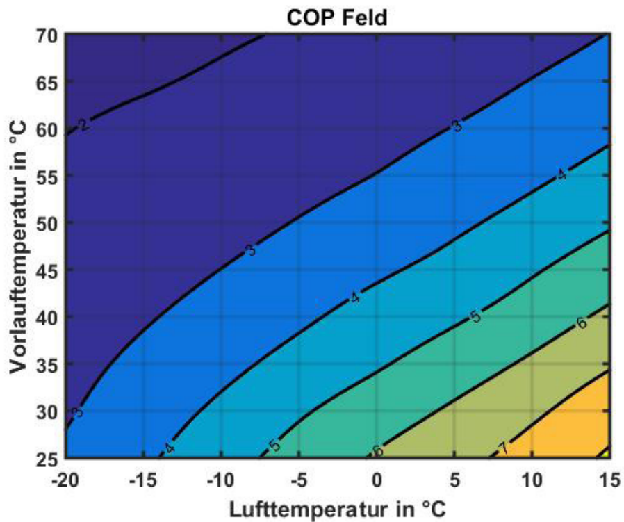
Abbildung 30: EU08L bei 6kW Heizleistung
