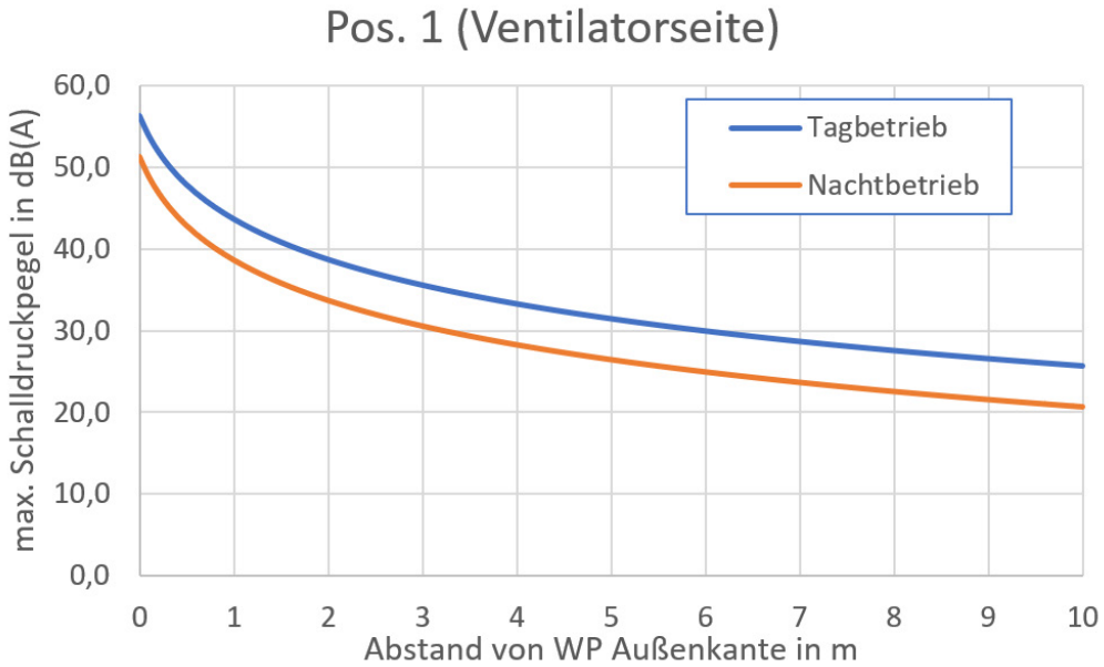
Abbildung 36: Schalldruckpegel EU13L, Vorderseite, freistehend
