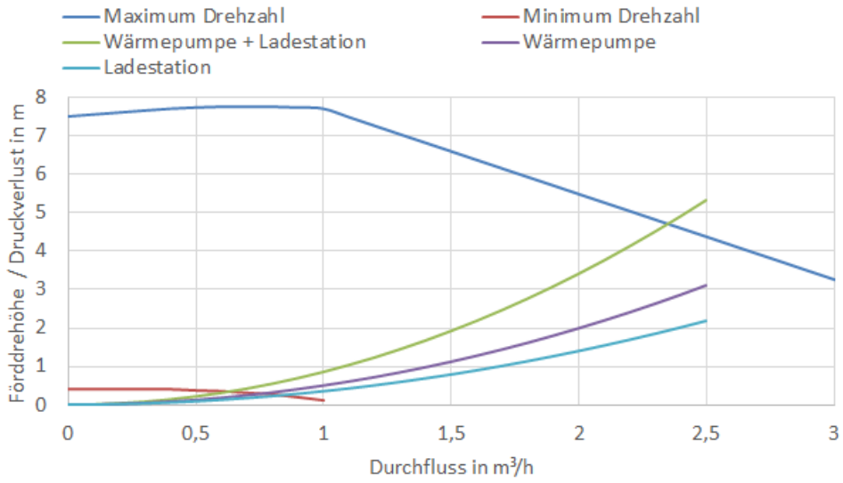
Abbildung 33: Pumpenkennlinie Grundfoss UPM3L 75/180 und Anlagenkennlinie
