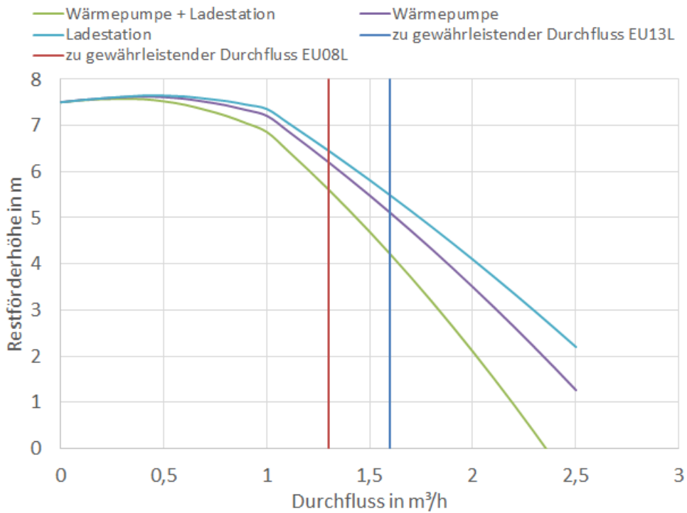
Abbildung 34: Restförderhöhe
