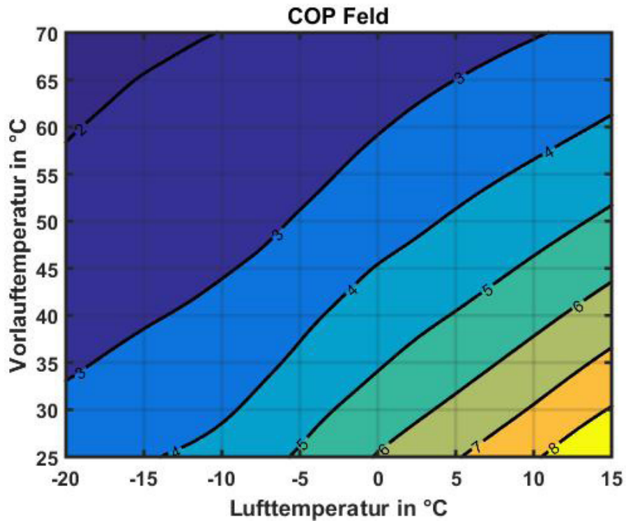
Abbildung 29: EU13L bei 9kW Heizleistung
