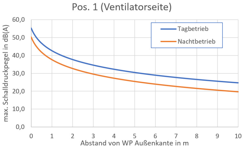
Abbildung 35: Schalldruckpegel EU08L, Vorderseite, freistehend
