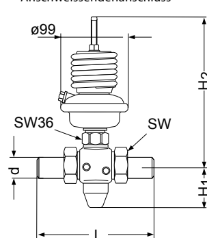
Anschweisendenanschluss
