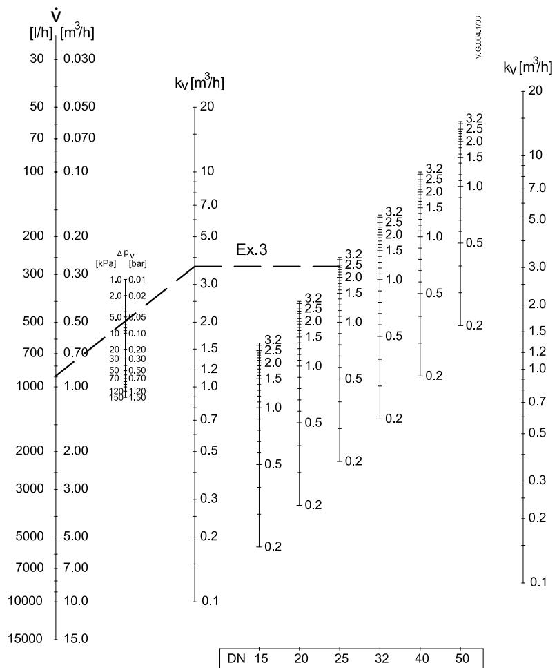
Abb. D: Dimensionierungsdiaqramm für das ASV-I, DN 15-50
