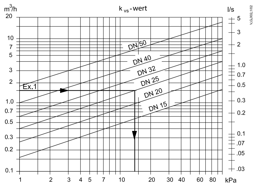
Abb. E: Druckabfall über dem ASV-M Ventil, DN 15-50
