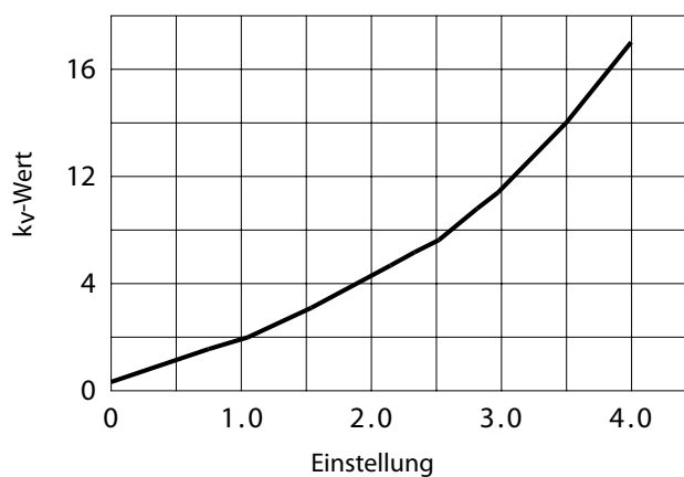
Durchflusscharakteristik
