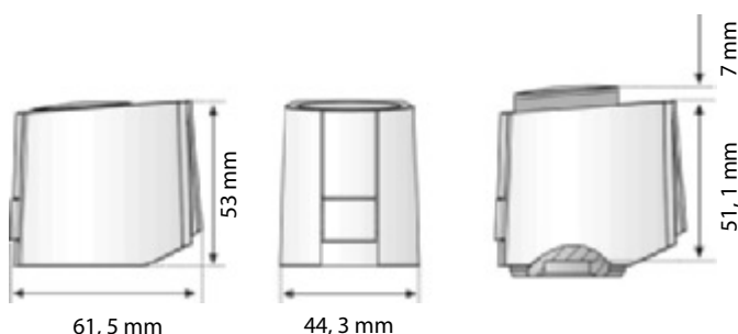
Abmessungen
