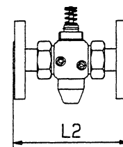
Flansch
