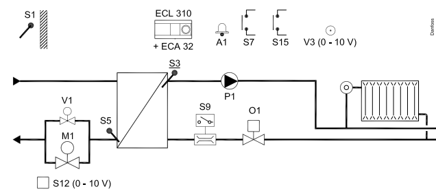
2 x MCV mit 0-bis-10-V- bzw. 3-Punkt-Regelung
