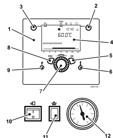
Abb.2 Bedienelemente
