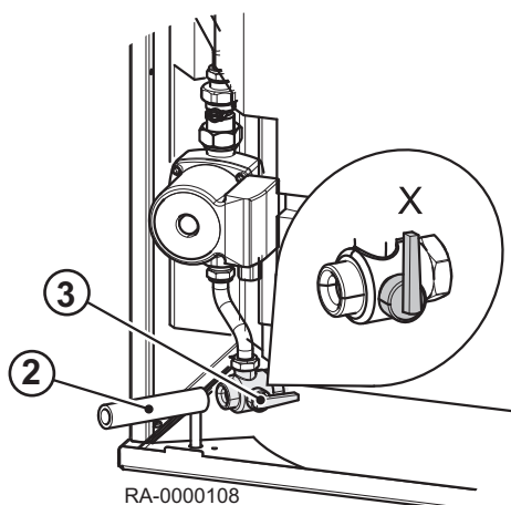
Abb.5 Entleeren des Speichers
