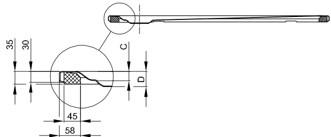
Darstellung mit vormontiertem Minimum-Wannenträger (T1).
