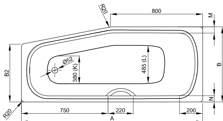
N° 2: Schräge Fußende rechts
