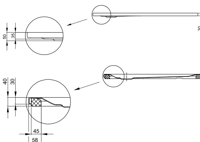
Darstellung mit vormontiertem Minimum-Wannenträger (T1).
