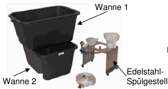
Abb. 1: Harzaustauschset HSS
