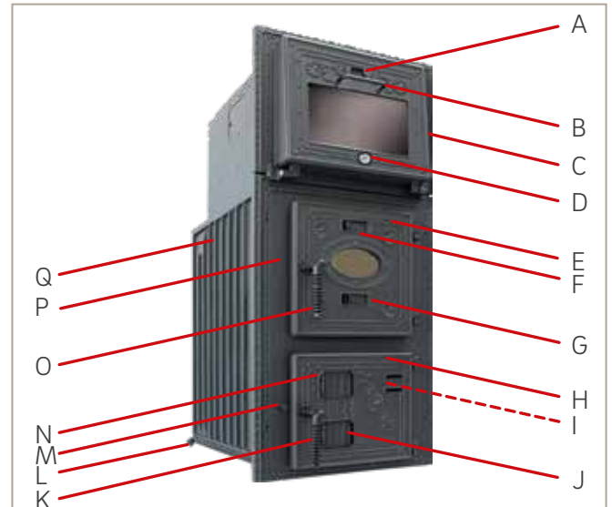
Abb. 8: JU 11 Soufflé
