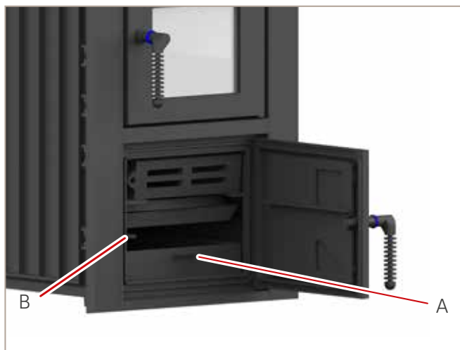
Abb. 17: Aschekasten entnehmen
