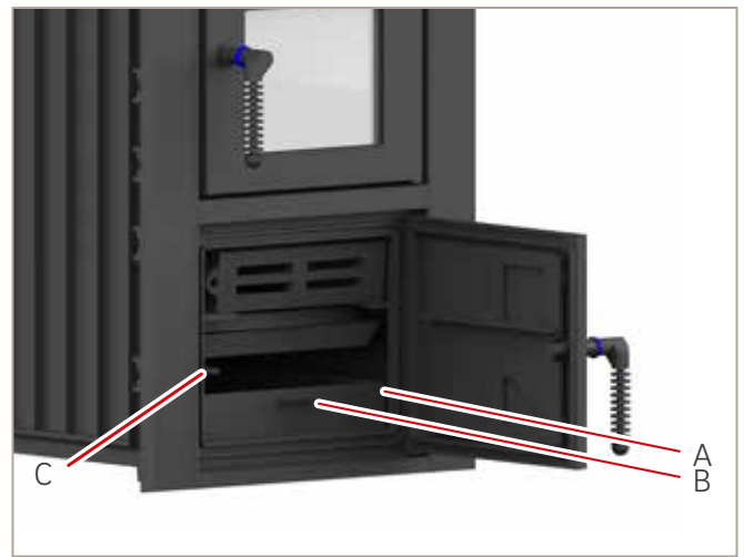
Abb. 28: Aschekasten entnehmen
