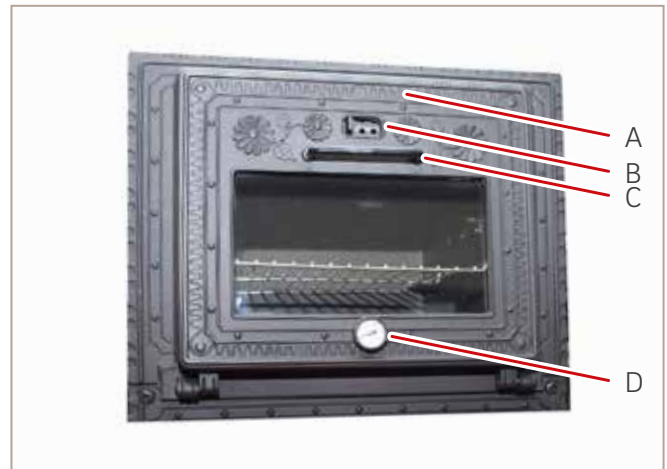
Abb. 21: Bedienelemente Soufflé
