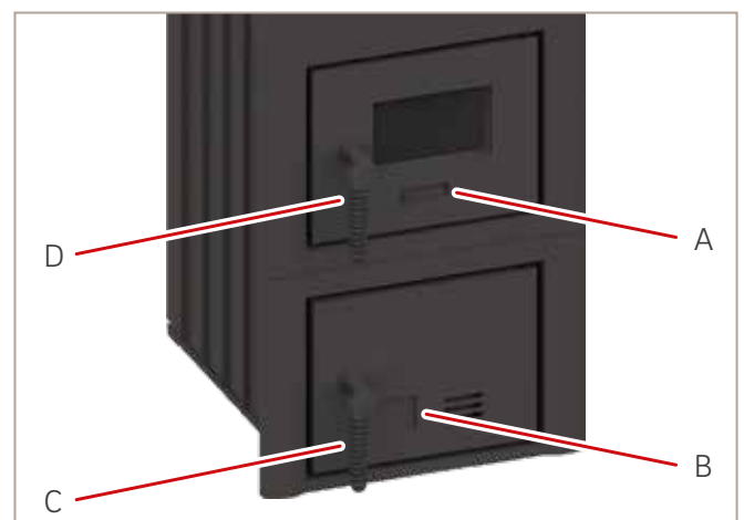
Abb. 15: Bedienelemente Format 6
