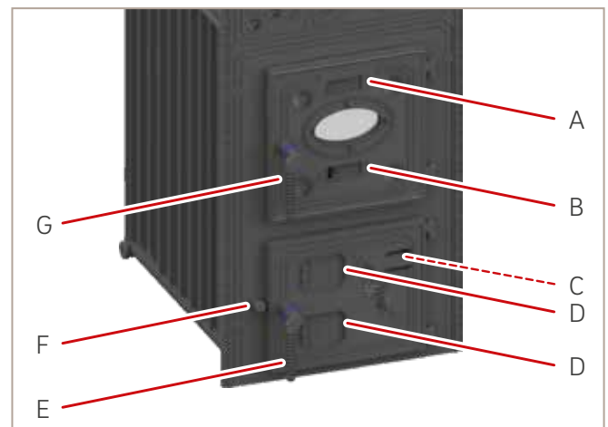
Abb. 18: Bedienelemente am Beispiel JU 11
