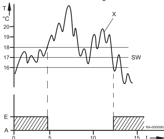
Abb.28 Sommer-/Winterheizgrenze
