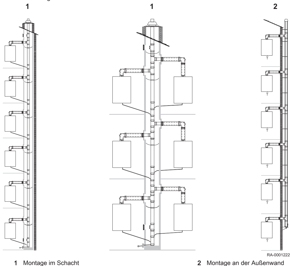
Abb.21 Montagearten
