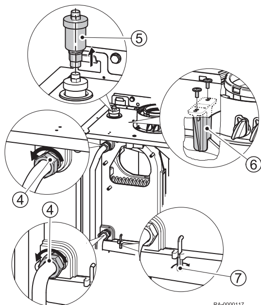
Abb.46 Wärmetauscher ausbauen
