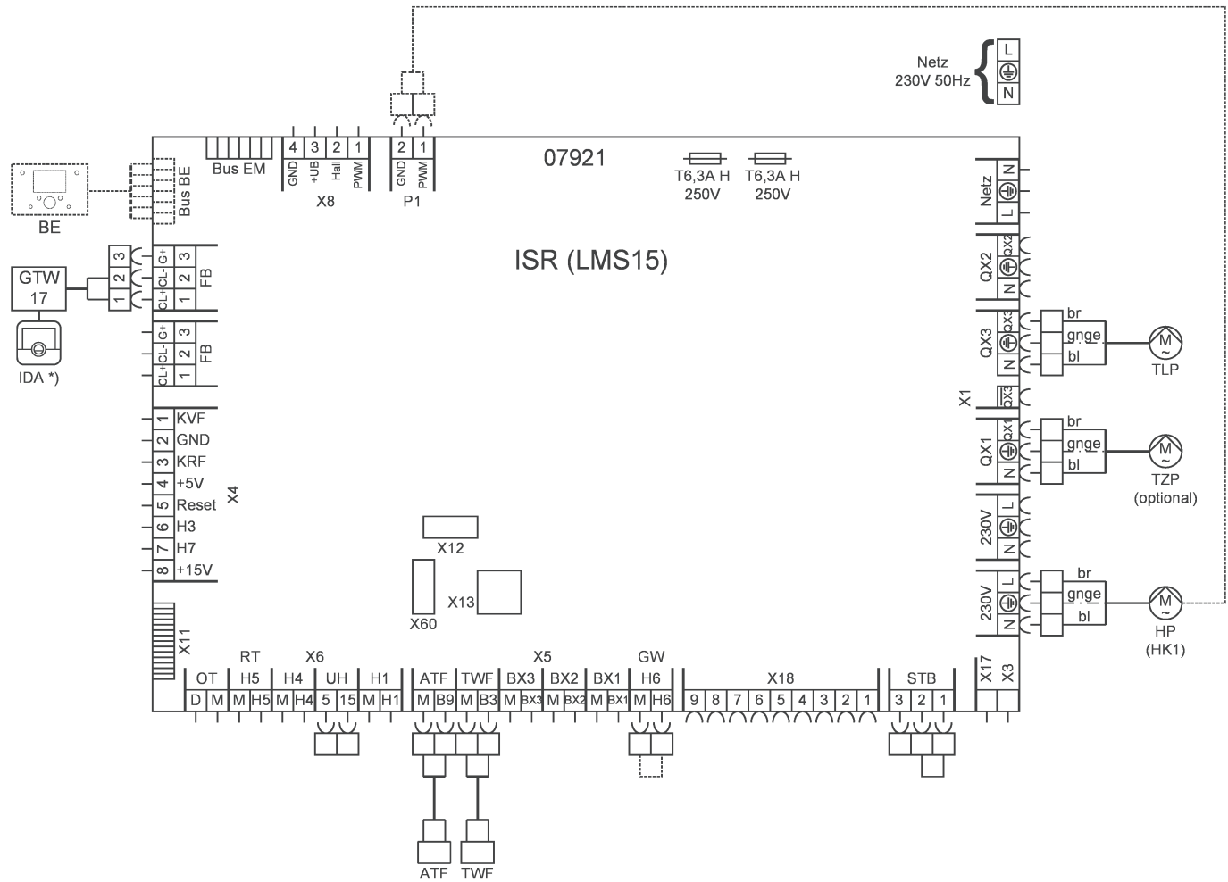
Abb.13 Anschlussplan
