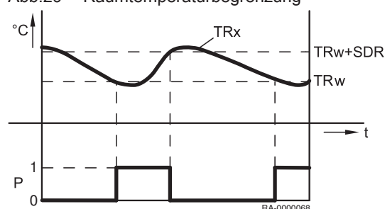
Abb.29 Raumtemperaturbegrenzung
