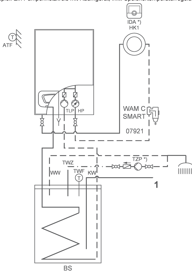
Abb.12 Anwendungsbeispiel: Ein Pumpenheizkreis mit Raumgerät, inkl. Speichertemperaturregelung
