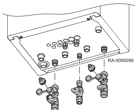
Abb.14 Einbau Absperrventile
