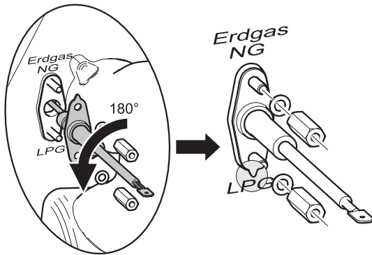
Abb.23 Umstellung auf Flüssiggas
