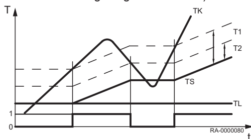
Abb.37 Laderegelung /schematisch)
