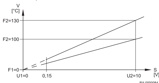
Abb.41 Beispiel für Wärmeeanforderung 10 V
