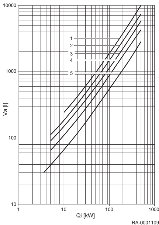
Abb.10 Anlagenvolumenbestimmung
