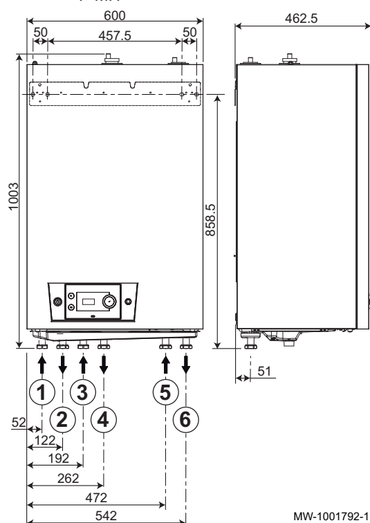
Abb.6 Mit Elektroheizeinsatz: BLW Mono-P MH
