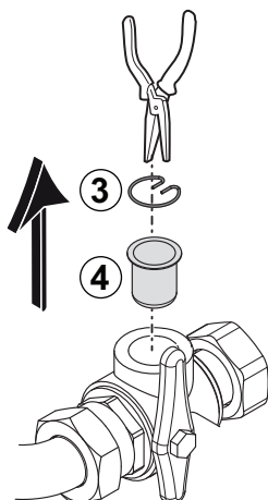
Abb.65 Sprengring und Filter herausnehmen
