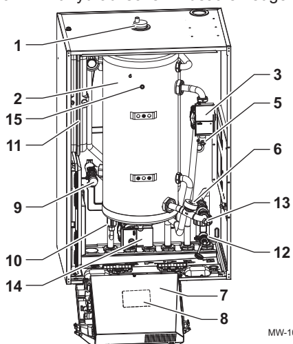
Abb.9 Mit hydraulischem Zusatzerzeuger
