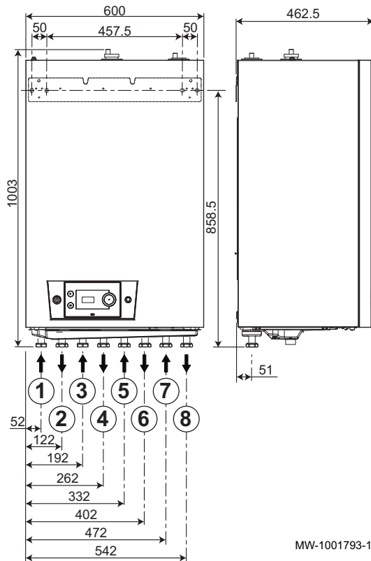
Abb.7 Ohne Elektroheizeinsatz: BLW Mono-P OH
