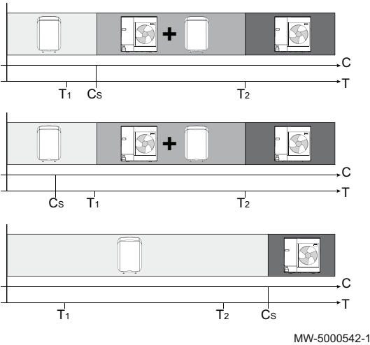
Abb.52 Einfluss von Außentemperaturen und Bivalenz.
