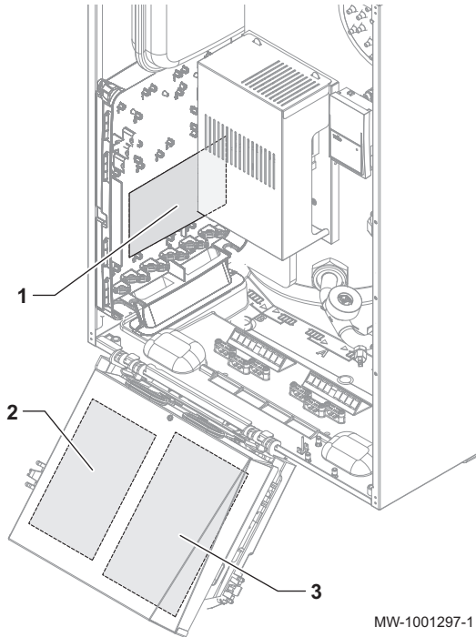
Abb.10 Position der Regelungsleiterplatten
