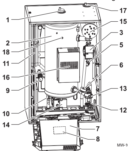
Abb.8 Mit elektrischem Zusatzerzeuger
