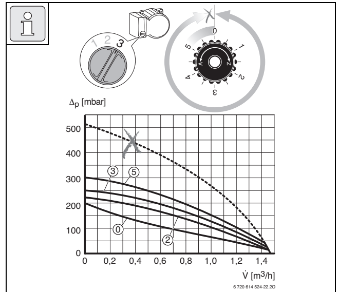
2.3 ZB 3/5-16 A, Z.B 7/11-22 A, ZWB 7/11-26 A
