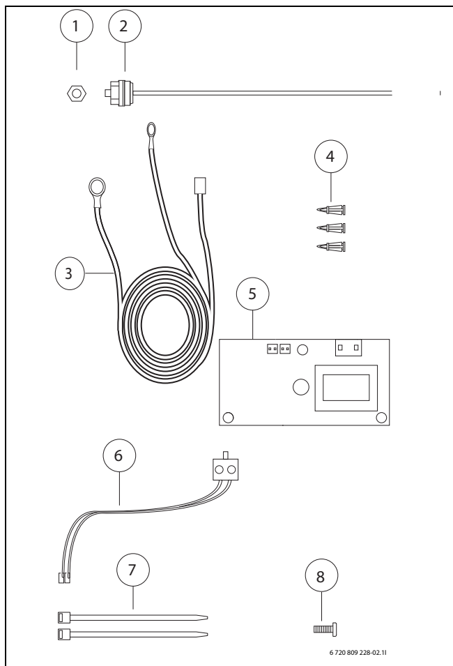
Рис. 19 Комплект поставки
