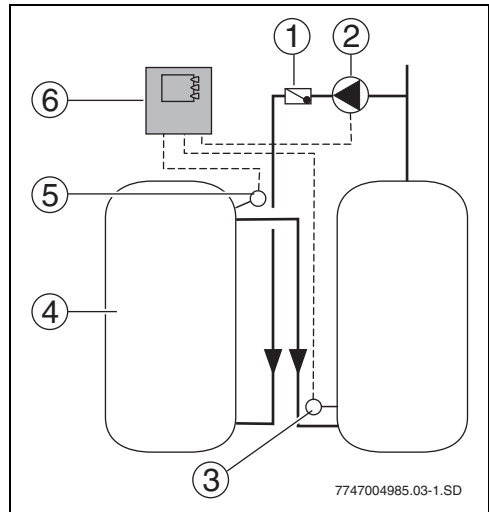
Bild 4 Umschichtfunktion
