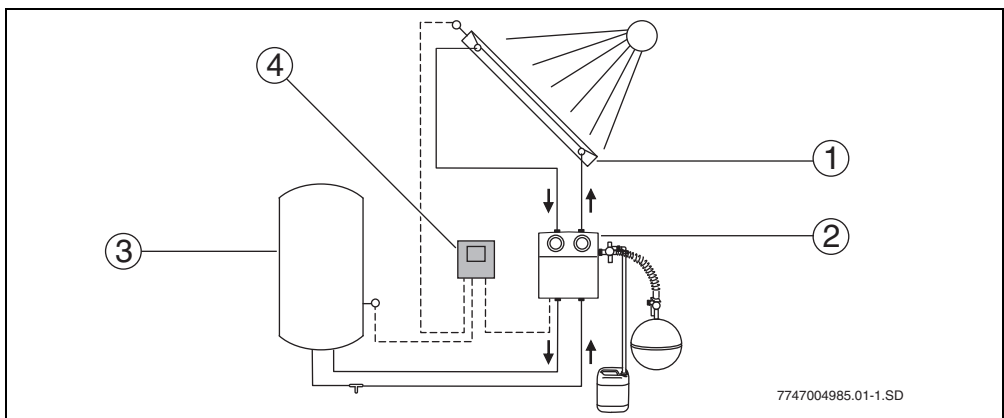
Bild 2 Anlagenschema
