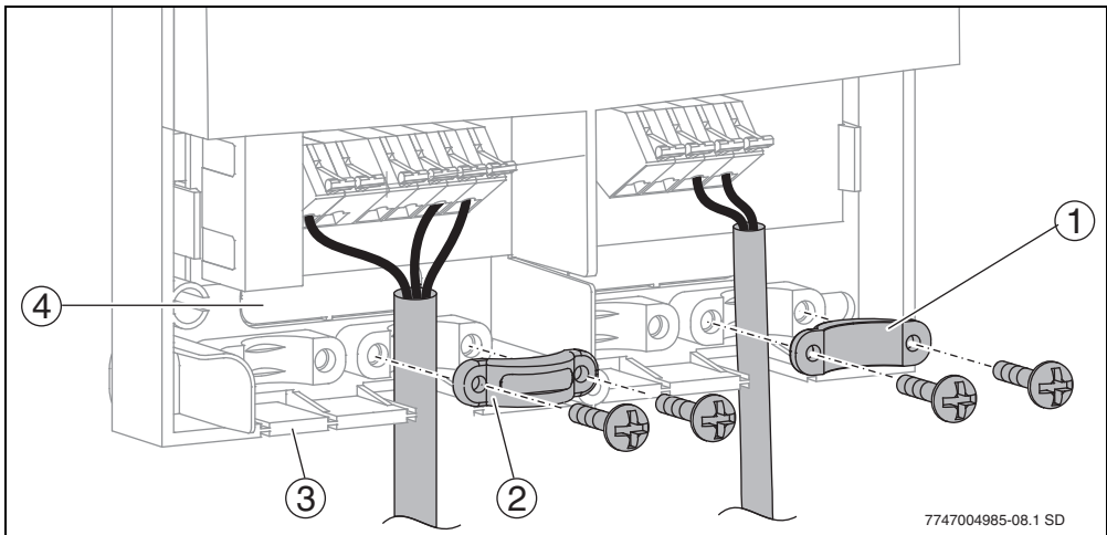
Bild 11 Durchführung und Befestigung der Kabel
