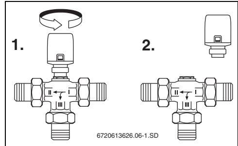
Bild 10 Stellantrieb demontieren
