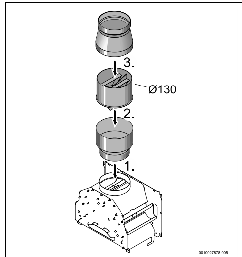
Bild 13 Ø 130 mm montieren
