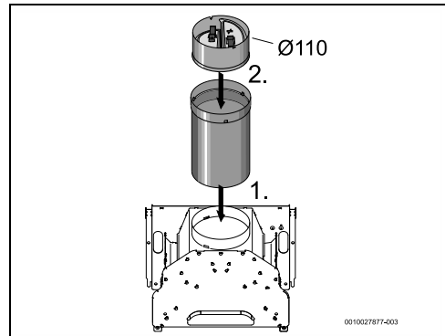
Bild 12 Ø 110 mm montieren
