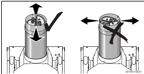
Bild 11 Abgasklappe montieren
