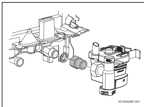
Fig. 45 Bague supplémentaire
