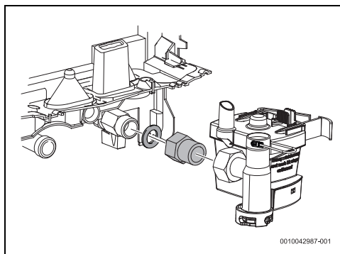
Rys. 70 Dodatkowa tuleja
