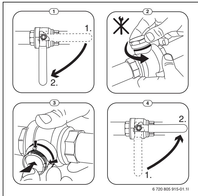
Bild 7 Siebreinigung
