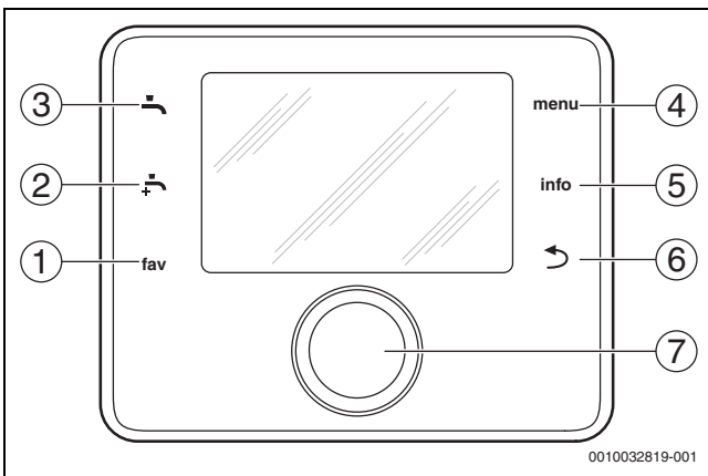
Bild 5 Bedienelemente
