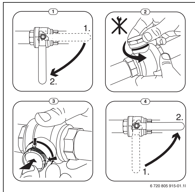
Bild 8 Siebreinigung
