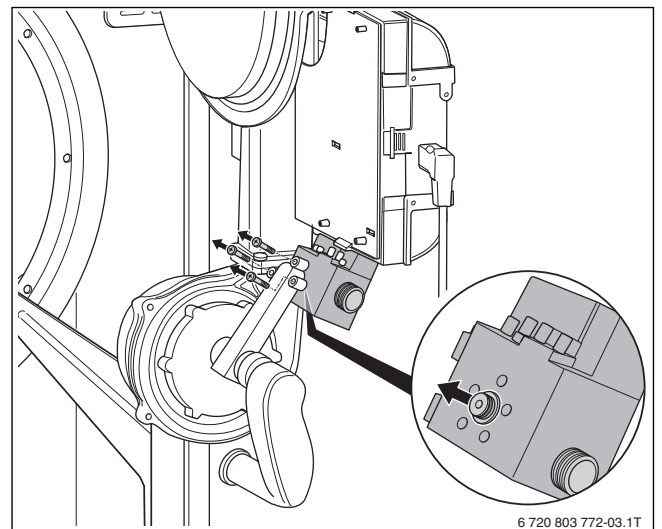
Rys. 12 Wymiana dyszy gazowej
