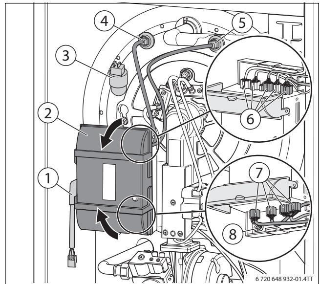
Fig. 3 Détacher les connexions à fiches
