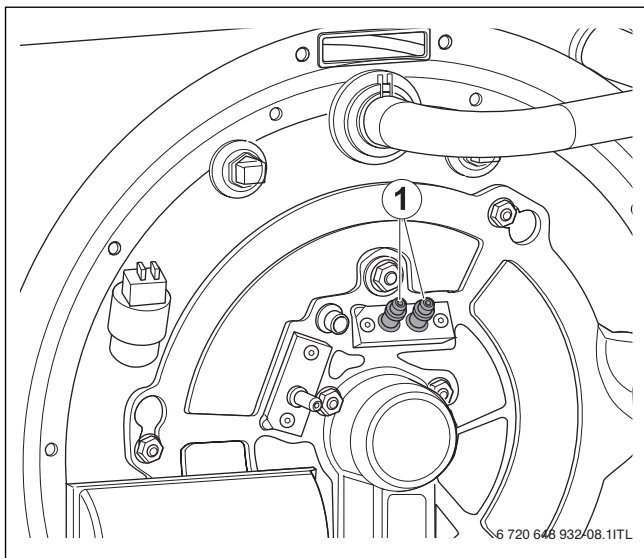
5. ábra Gyújtóelektróda
