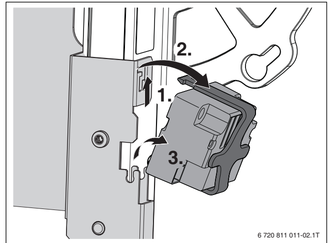
Fig. 6 Retirar el transformador de encendido
