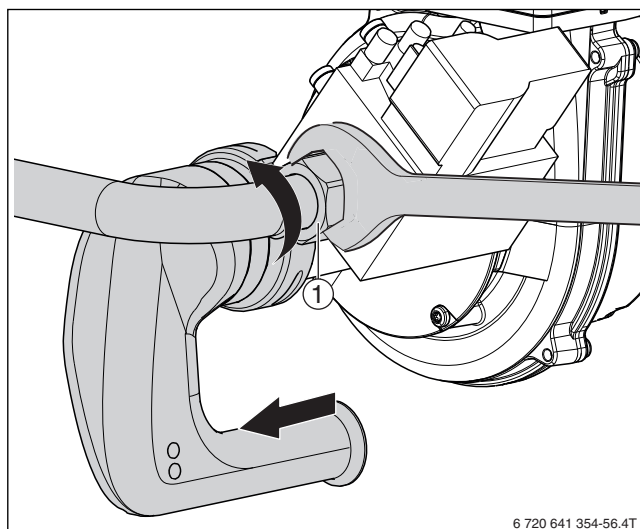
Fig. 8 Soltar as uniões rosca no dispositivo de controle do gás (imagem exemplificativa da caldeira de 22 kW)
