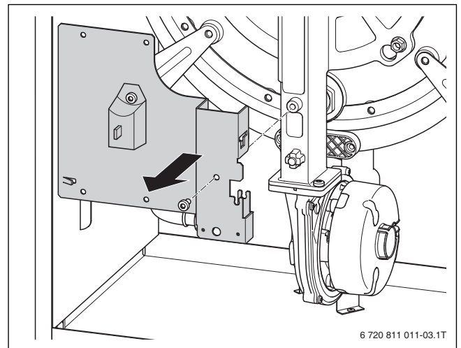
Fig. 7 Desmontar chapa deflectora
