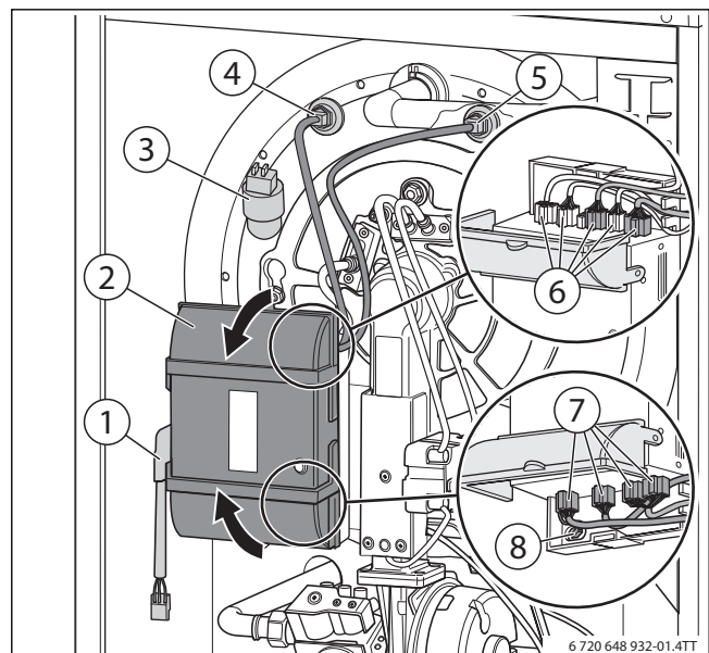
Afb. 3 Steekverbindingen losmaken
