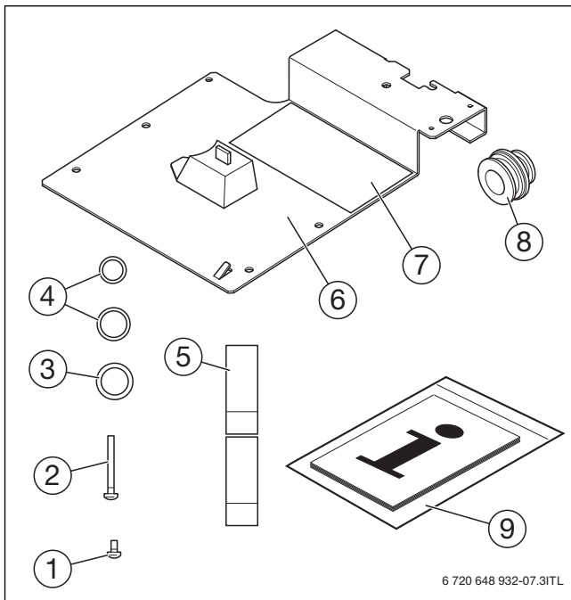
Afb. 1 Leveringsomvang
