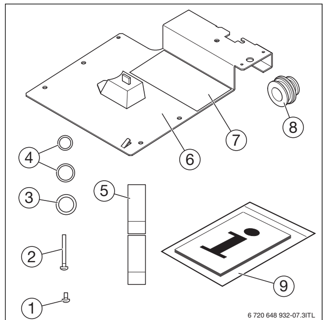
Obr. 1 Rozsah dodávky
