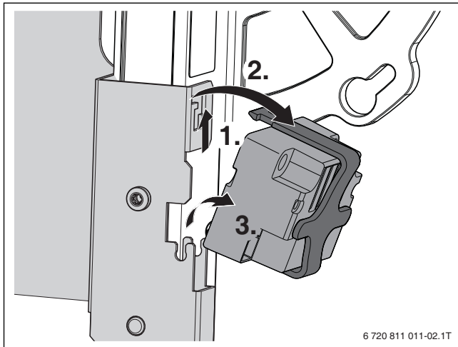
Bild 6 Zündtrafo entnehmen
