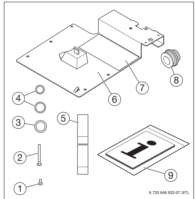
Rys. 1 Zakres dostawy
