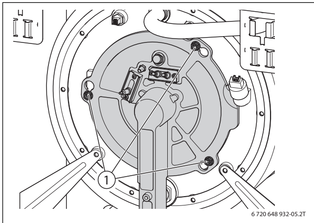
Afb. 10 Bevestigingsmoeren losdraaien
