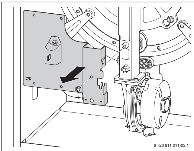
Bild 7 Halteblech demontieren
