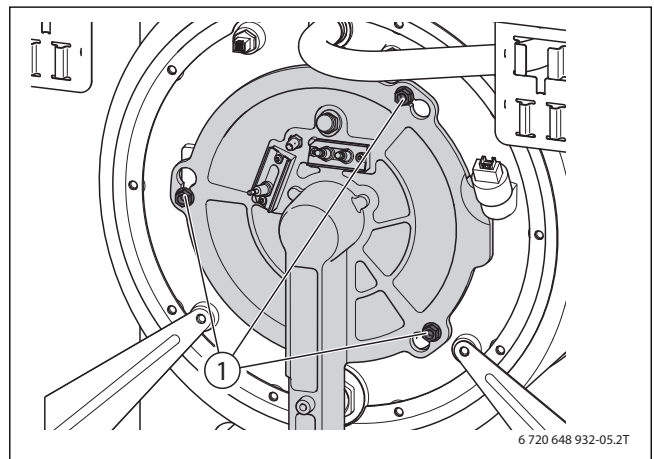
Obr. 10 Uvoľnenie upevňovacích matic
