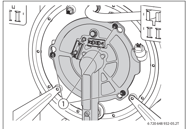
Bild 10 Befestigungsmuttern lösen
