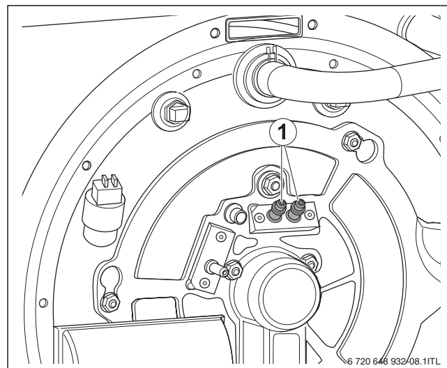
Obr. 5 Zapalovacia elektróda
