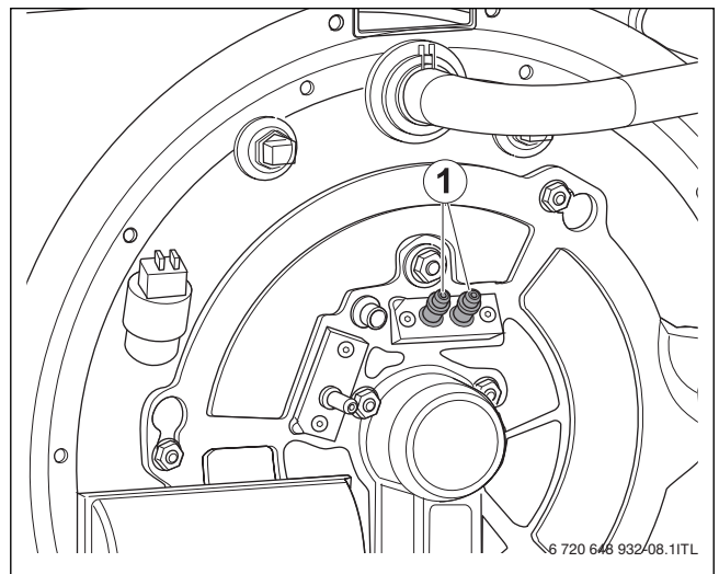
Fig. 5 Electrode d'allumage
