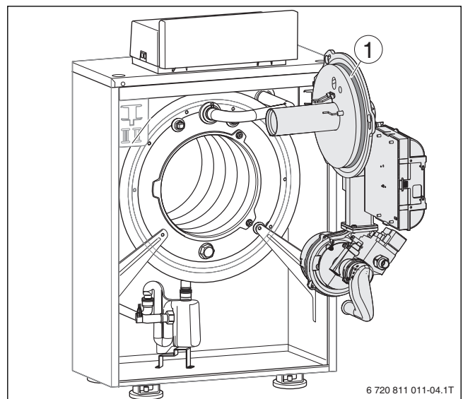
Afb. 13 O-ring branderhuis
