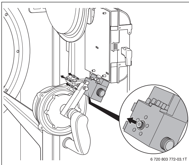
Afb. 12 Inspuiter vervangen
