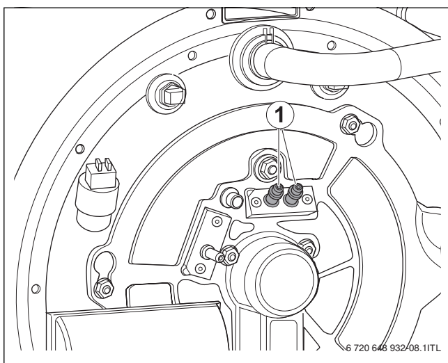
Afb. 5 Ontstekingselektrode
