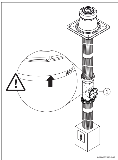
7 Ø 110: 7738112696
