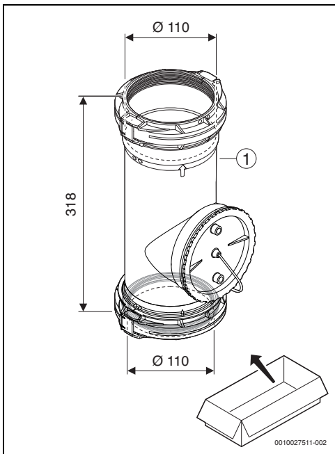
3 \text{Ø}110 : 7738112696
