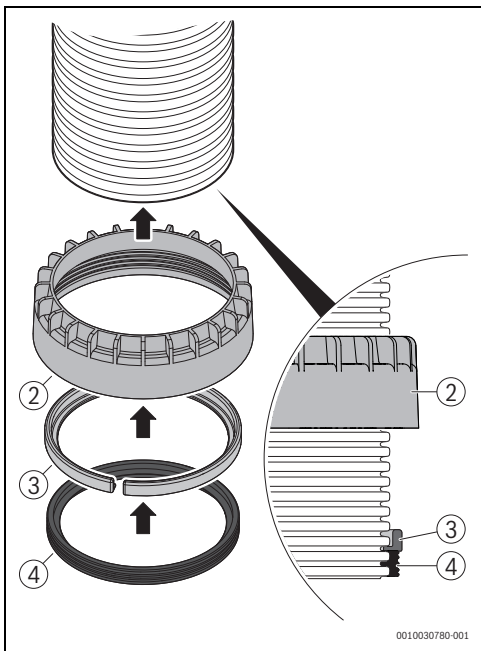
11 Ø 80: 7738112692
