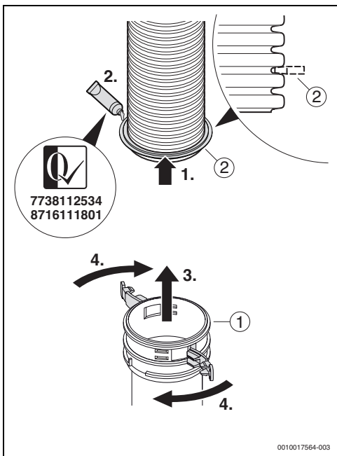
9 Ø 60: 7738112633
