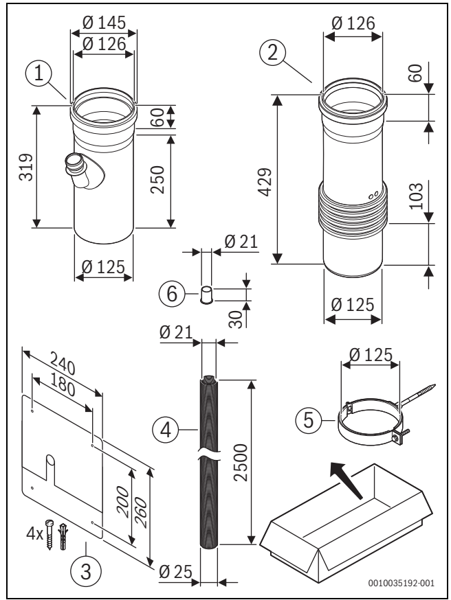
2 Ø125: 7738113346
