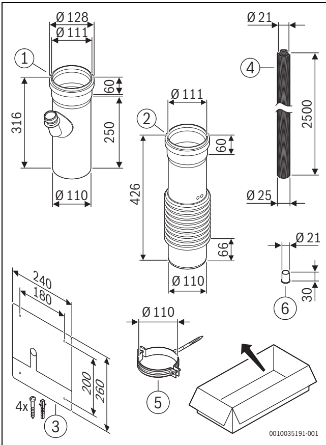
1 Ø110: 7738113345
