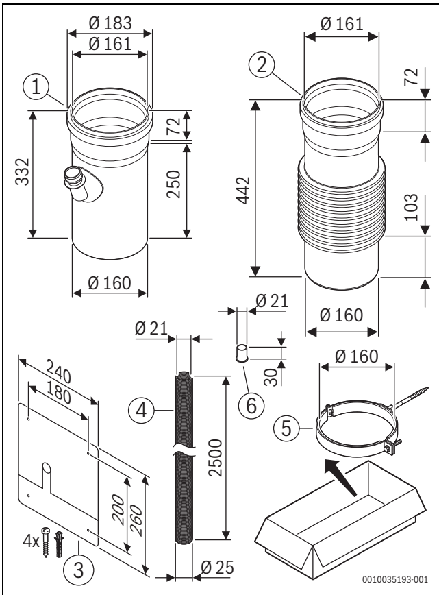
3 Ø160: 7738113347
