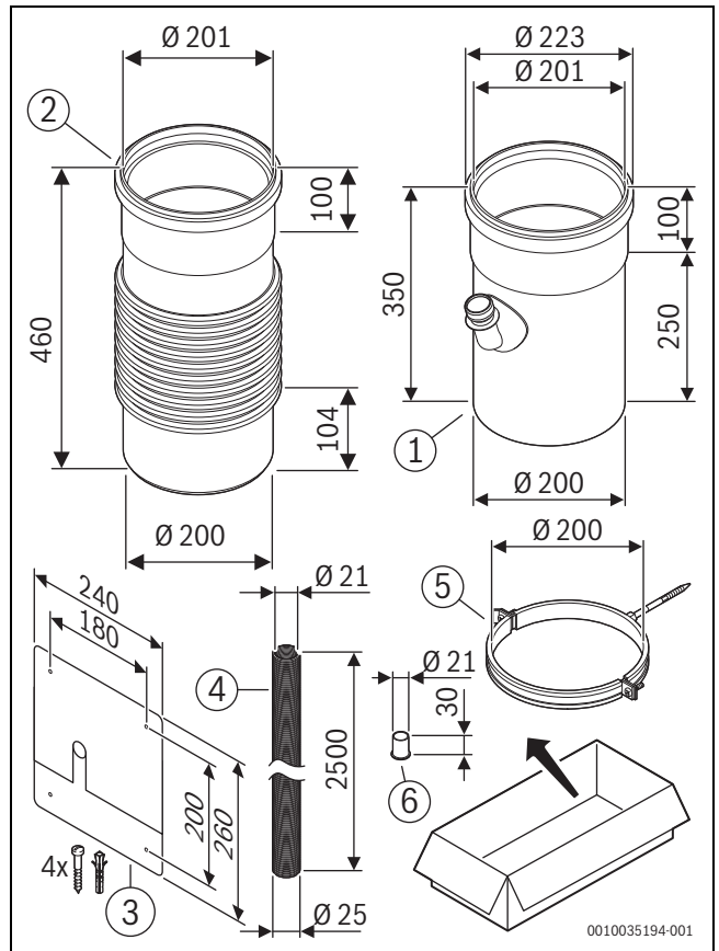
4 Ø200: 7738113348
