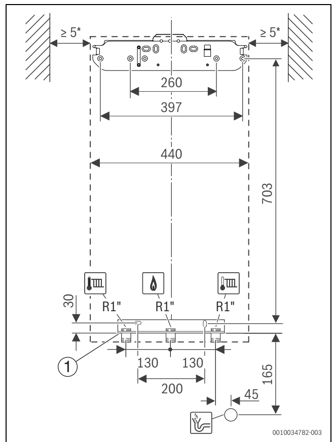
Bild 3 Frontansicht (mm)
