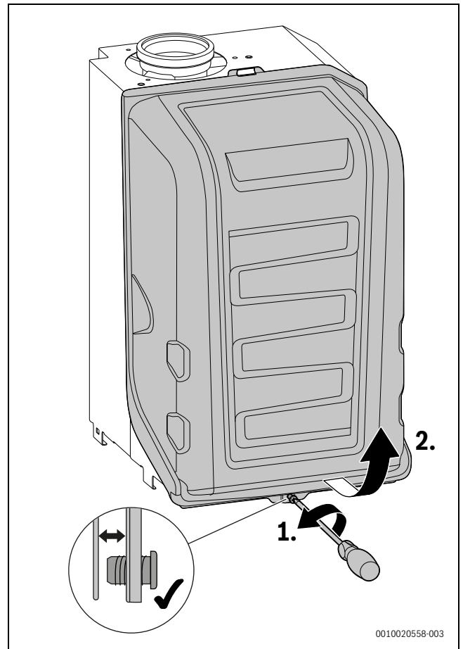
Bild 50 Brennerhaube abnehmen
