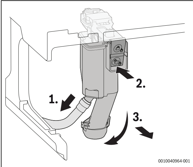
Bild 68 Kondensatsiphon ausbauen
