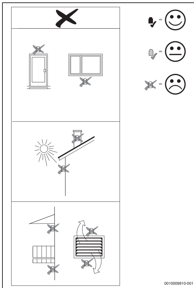
Bild 34 Ungeeigneter Installationsort des Außentemperaturfühlers
