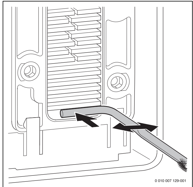
Bild 67 Kondensatwanne reinigen
