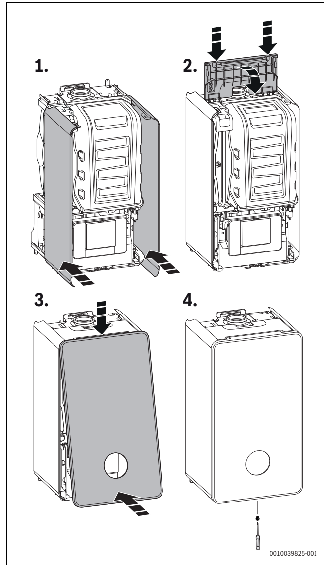
Bild 47 Verkleidung montieren
