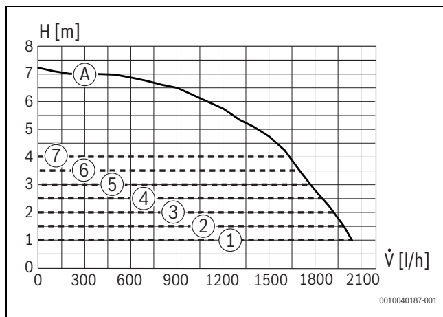
Bild 78 GC9800iW 50 H: Pumpenkennfelder und Pumpenkennlinien
