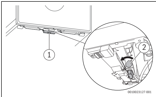
Bild 45 Connect-Key sichern
