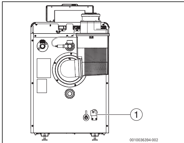
Bild 29 Haltewinkel montieren
