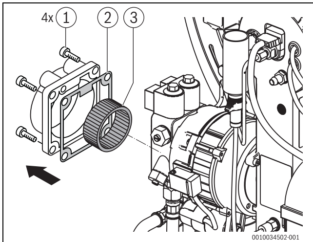
Bild 71 Ölpumpenfilter prüfen
