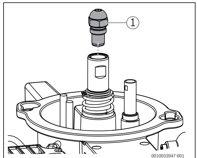
Bild 62 Düse abschrauben
