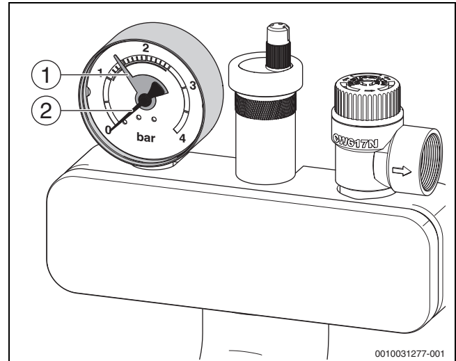
Bild 79 Manometer
