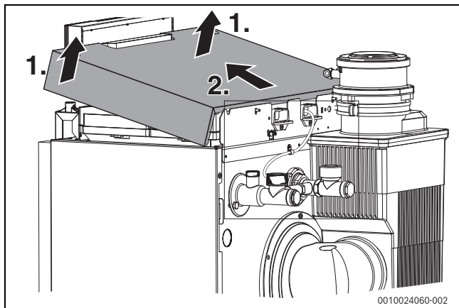
Bild 32 Kesselhaube abnehmen
