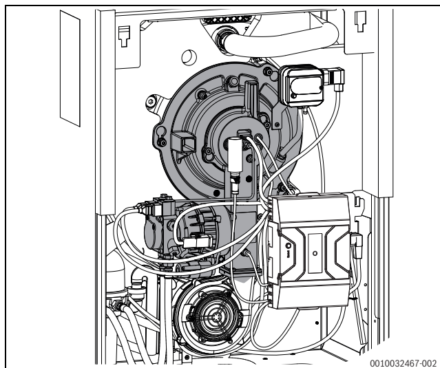
Bild 50 Heiße Bauteile am Brenner/Wärmetauscher
