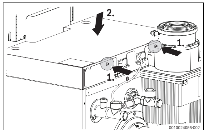
Bild 36 Kesselhaube montieren
