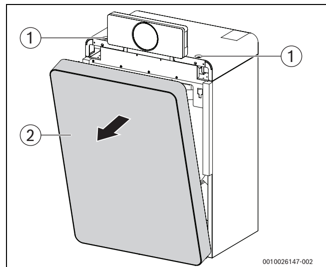
Bild 11 Kesselvorderwand demontieren
