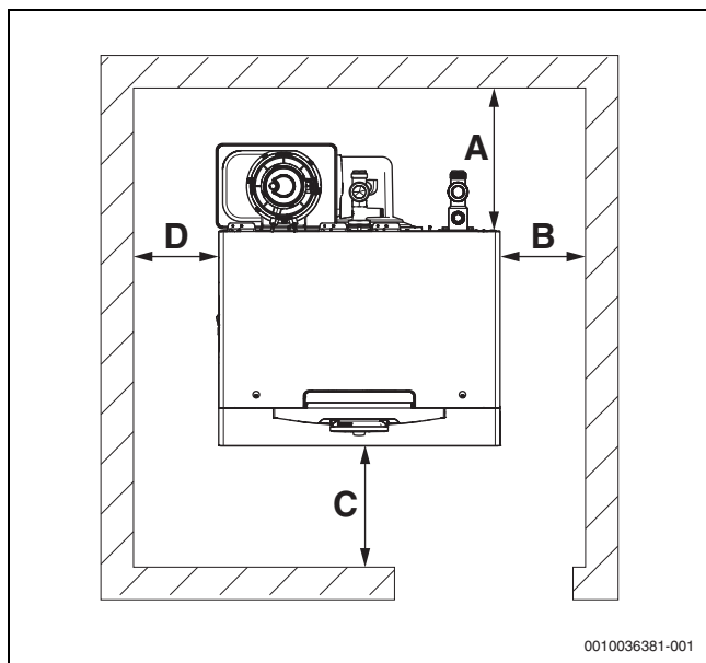
Bild 12 Wandabstände im Aufstellraum
