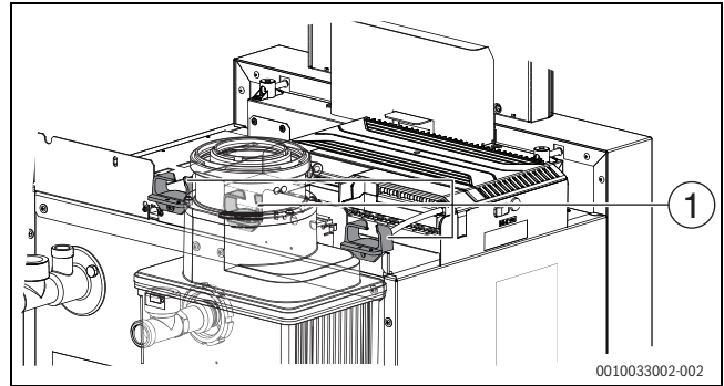
Bild 34 Kabel verlegen
