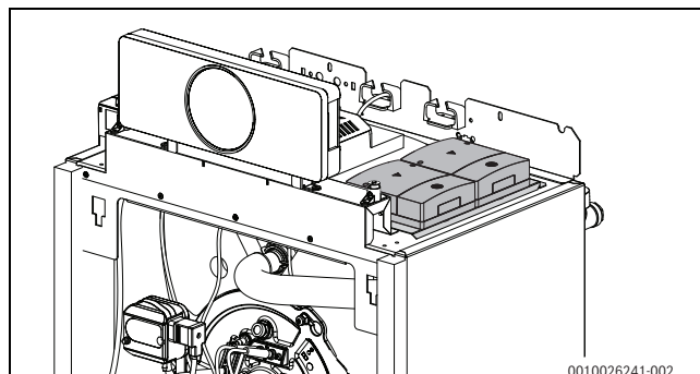
Bild 39 Standard-Funktionsmodule montiert
