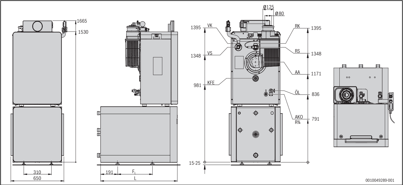
Bild 7 Abmessungen und Anschlüsse OC8800i F mit WH ...-3 P 2 B (Maße in mm)
