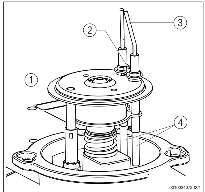
Bild 61 Mischsystem ausbauen
