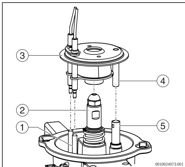
Bild 65 Mischsystem montieren
