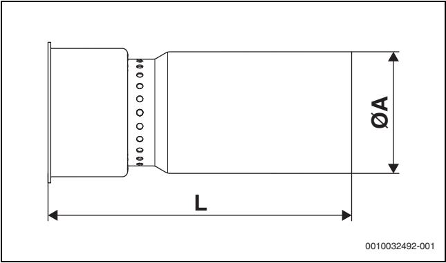
Bild 92 Brennerrohre
