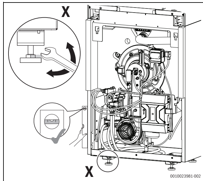
Bild 14 Heizkessel ausrichten
