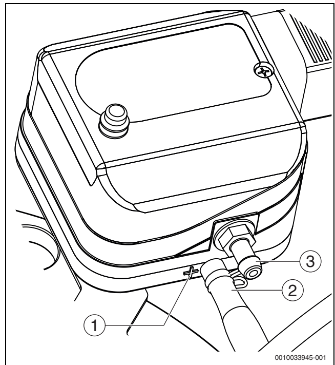
Bild 88 Detailansicht Druckwächter
