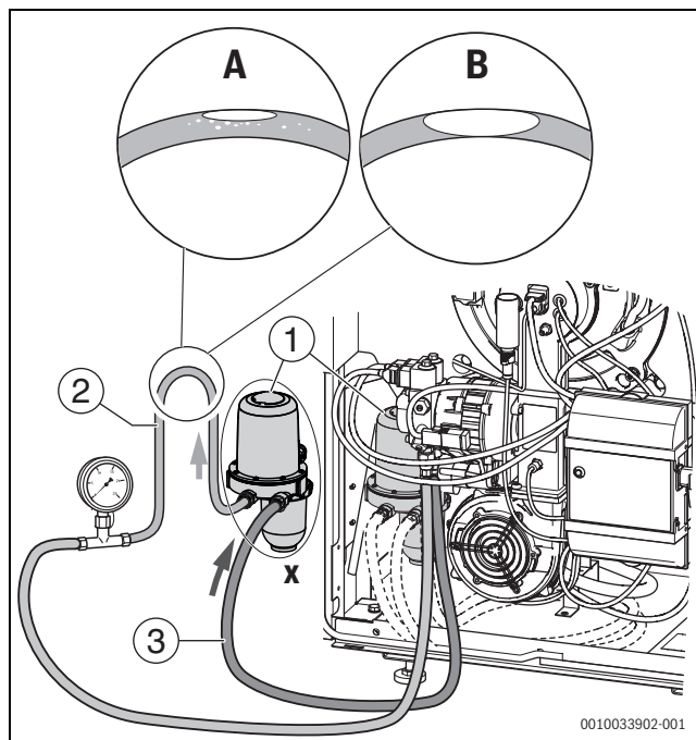
Bild 48 Dichtheit der Saugleitung prüfen
