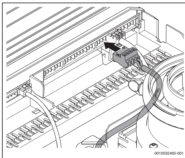
Bild 21 Kesselsicherheitsgruppe einstecken
