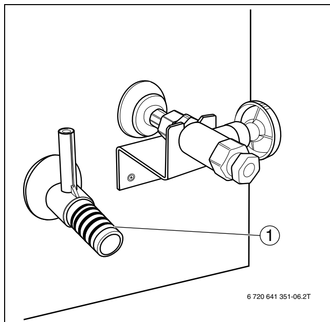
Bild 18 Anschluss Kondensatschlauch (dargestellt OC8800i F 19/25)
