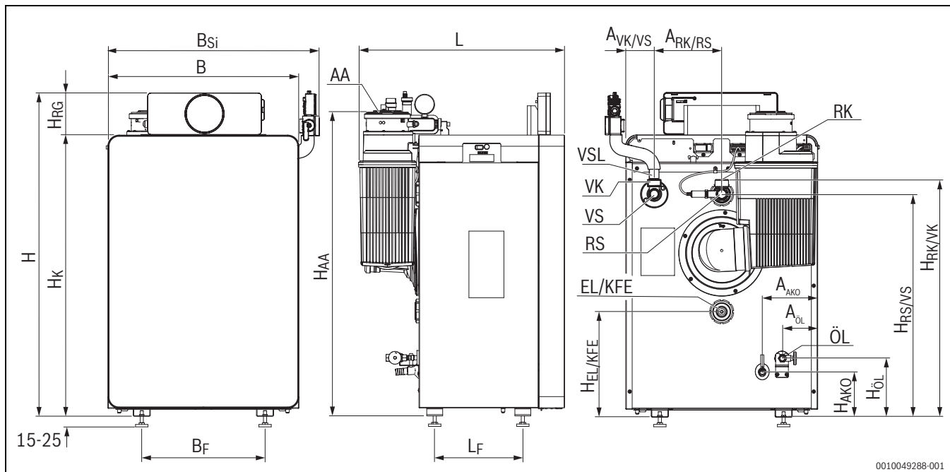
Bild 6 Anschlüsse und Abmessungen für OC8800i F 19/25 (Maße in mm)
