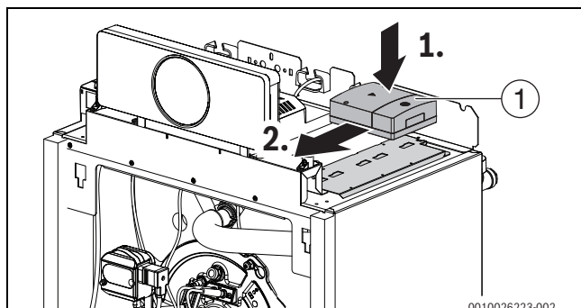
Bild 38 Funktionsmodule einstecken
