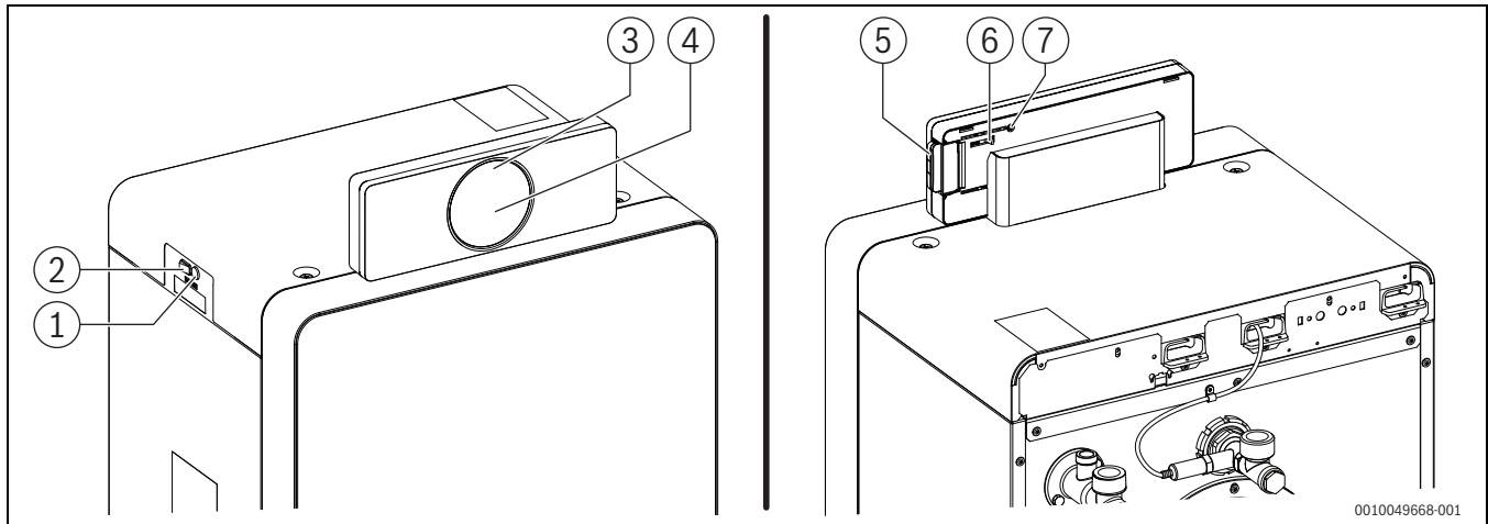
Bild 5 Regelgerät IMX35 mit Bedienfeld UI800
