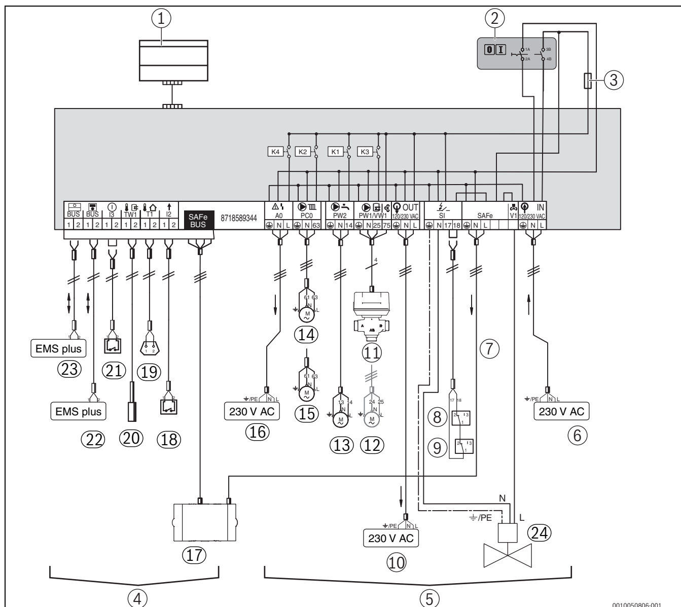
Bild 89 Anschlussplan Regelgerät IMX35i
