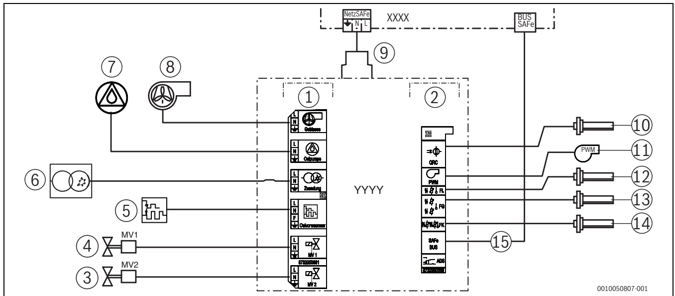
Bild 90 Anschlussplan digitaler Feuerungsautomat
