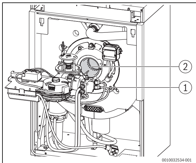
Bild 64 Dichtung prüfen (Serviceposition 2)
