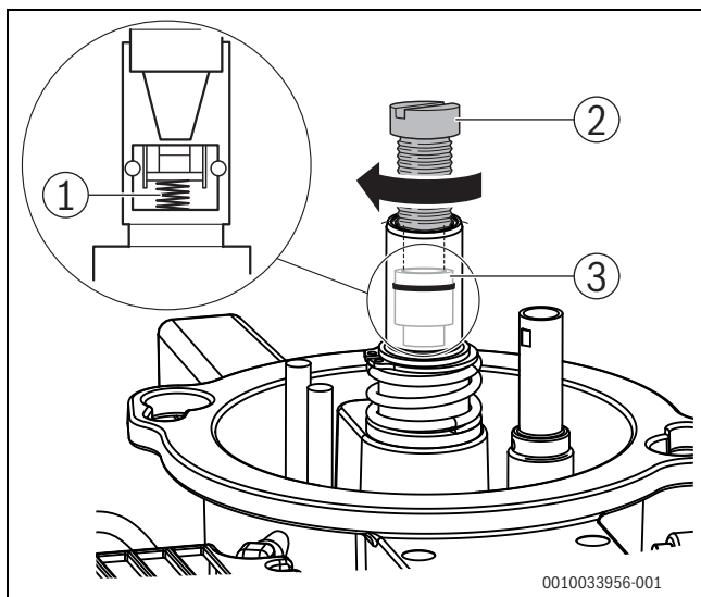
Bild 63 Abschlussventil austauschen
