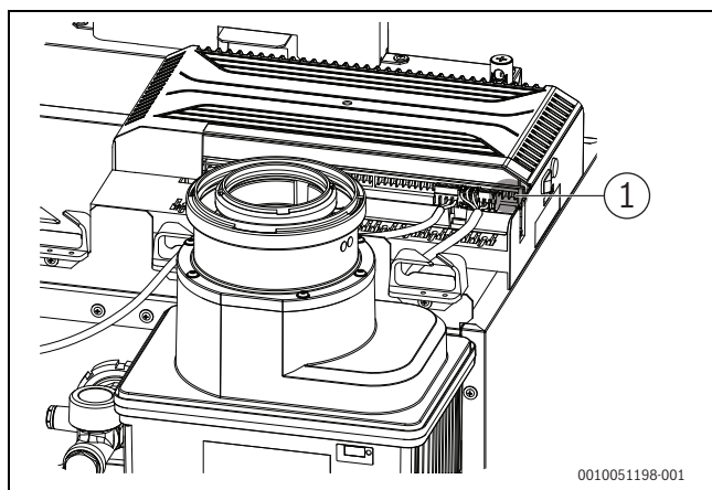
Bild 37 Netzanschluss herstellen
