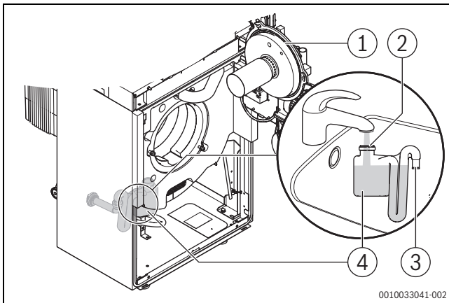
Bild 78 Siphon reinigen
