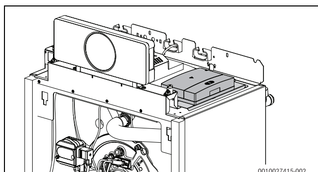
Bild 40 Großes Funktionsmodul montiert
