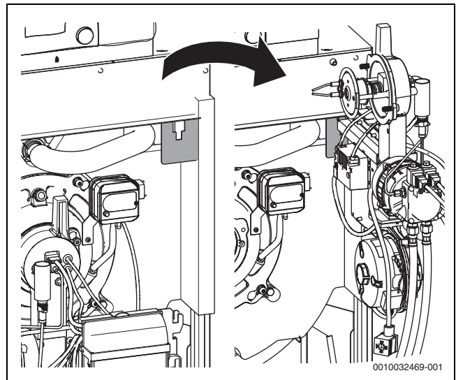
Bild 59 Brenner in Serviceposition 1 einhängen
