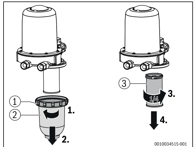
Bild 73 Filtertasse entfernen
