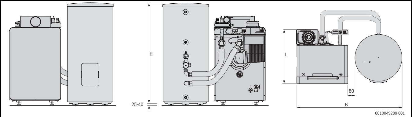
Bild 8 Abmessungen und Anschlüsse OC8800i F mit W ...-5 P1 A (Maße in mm)
