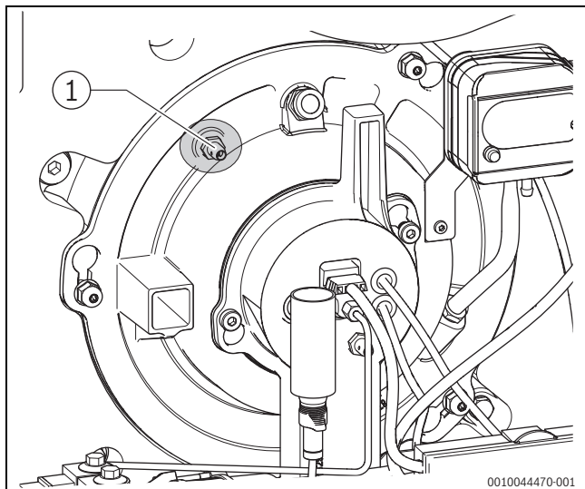
Bild 74 Druckmessstelle am Brenner
