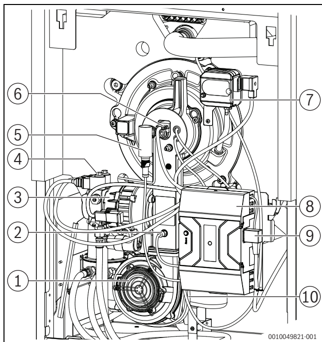
Bild 2 Ölbrenner
