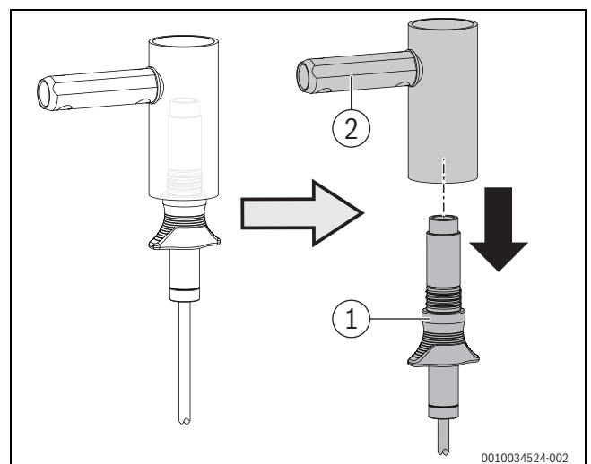
Bild 81 Flammenfühler demontieren
