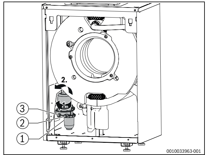
Bild 72 Ölfilter demontieren
