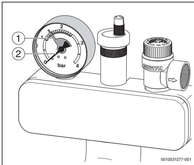
Bild 24 Manometer (Beispiel)
