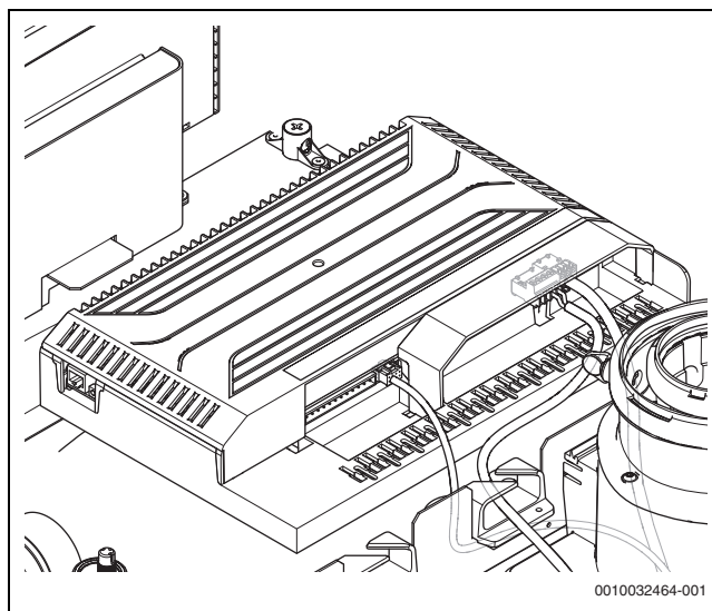
Bild 20 Gehäuseklemmenabdeckung abnehmen
