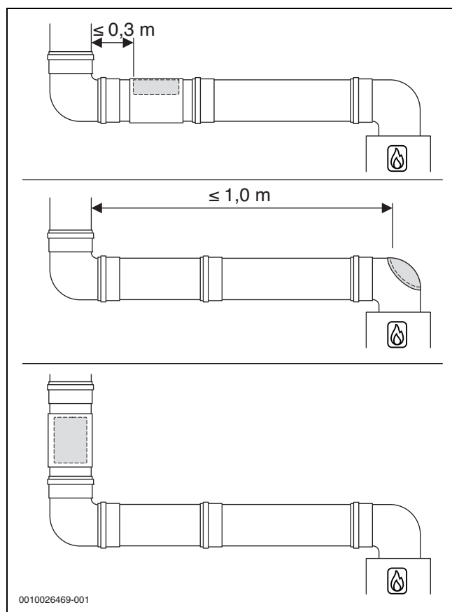
Bild 1 Anordnung der unteren Prüfoffnung
