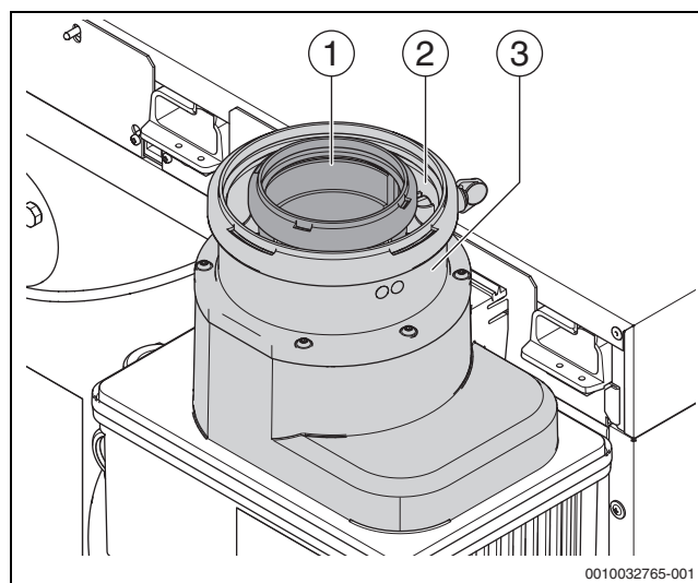
Bild 15 Abgasanschluss montieren
