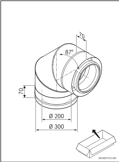
2 FC-CE200-87: 7746900984
