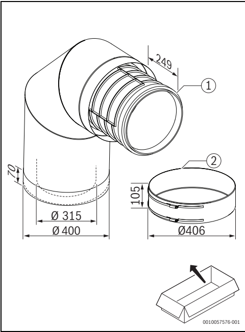
4 FC-CE315-87: 7738114045
